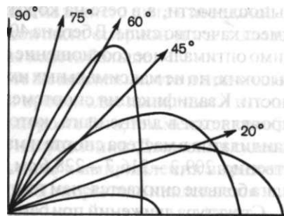
Рис. 184. Зависимость между направлением силы толчка и траекторией центра тяжести "Р" полете
