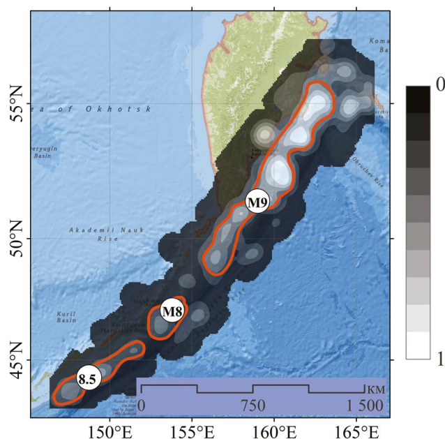
Рис. 9. Объединенная карта плотности независимых и связанных событий. Оранжевые линии очерчивают контуры, соответствующие областям разрыва потенциальных сильнейших землетрясений Курило-Камчатской дуги с магнитудами 8, 8.5 и 9.
