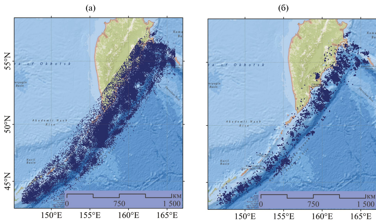
Рис. 5. Независимые (а) и связанные (б) землетрясения, полученные после объединения двух каталогов (удаления дубликатов) и последующей декластеризации полученного объединенного каталога.
