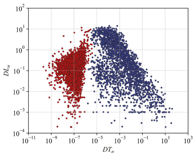
Рис. 3. Пространственно-временная структура результатов идентификации дубликатов, где DT_\sigma = DT/\sigma_T , DL_\sigma = \sqrt{\frac{DX^2}{\sigma_X^2} + \frac{DY^2}{\sigma_Y^2}} . Красным цветом показаны события, идентифицированные как дубликаты, синим — связанные события.
