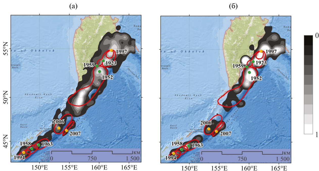
Рис. 6. Карты плотности количества независимых (а) и связанных (б) землетрясений в сопоставлении с областями разрыва (красные линии) сильнейших землетрясений ( M \geq 7.8 ) Курило-Камчатской дуги из табл. 2. Эпицентры землетрясений до 1990 г. отмечены зелеными точками, после 1990 г. — желтыми точками. Цифрами обозначен год события.
