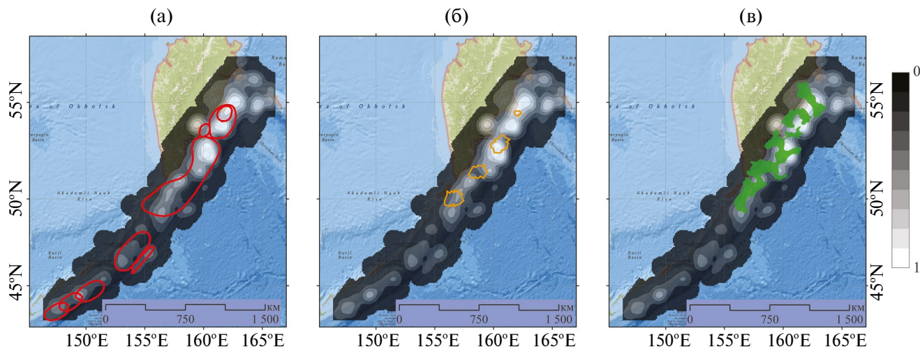
Рис. 8. Объединенная карта плотности количества событий в сопоставлении с моделями “асперити” для Курило-Камчатской зоны субдукции: (а) модель 1 [Johnson, Satake, 1999; Burgmann et al., 2005; Rhea et al., 2010], линии красного цвета; (б) модель 2 [Burgmann et al., 2005], линии желтого цвета; (в) модель 3 [Vorobieva et al., 2018], области зеленого цвета.
