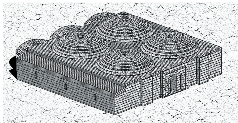
Илл. 3. Баня-тахаратхана («Дом феодала»). Вариант реконструкции здания, раскоп XVII (по Э. Д. Зиливинской).
