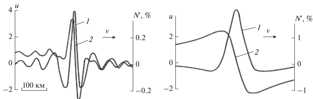
Рис. 2. Профили ВГВ в дальней зоне от очага и возбуждаемых ими в ионосфере ПИВ электронной концентрации при y = 0 : 1 – ВГВ; 2 – ПИВ ( N' ) при \varepsilon = -1.2 (слева) и \varepsilon = -12 (справа).
