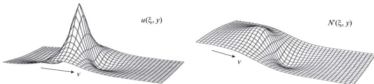
Рис. 1. Сейсмообусловленное ВГВ-возмущение в F -области ионосферы солитонного типа ( u ) при \varepsilon = -12 и соответствующее ему возмущение N' = \{[N_e(u, t) - N_e(0, t)]/N_e(0, t)\} \times 100\% .
