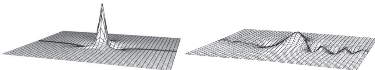
Рис. 3. Эволюция в F -области ионосферы возбужденного рэлеевской волной солитона ВГВ с учетом диссипативных эффектов ( \sigma = 1 ) при \varepsilon = -1.2 : t = 0, 0.2 .
