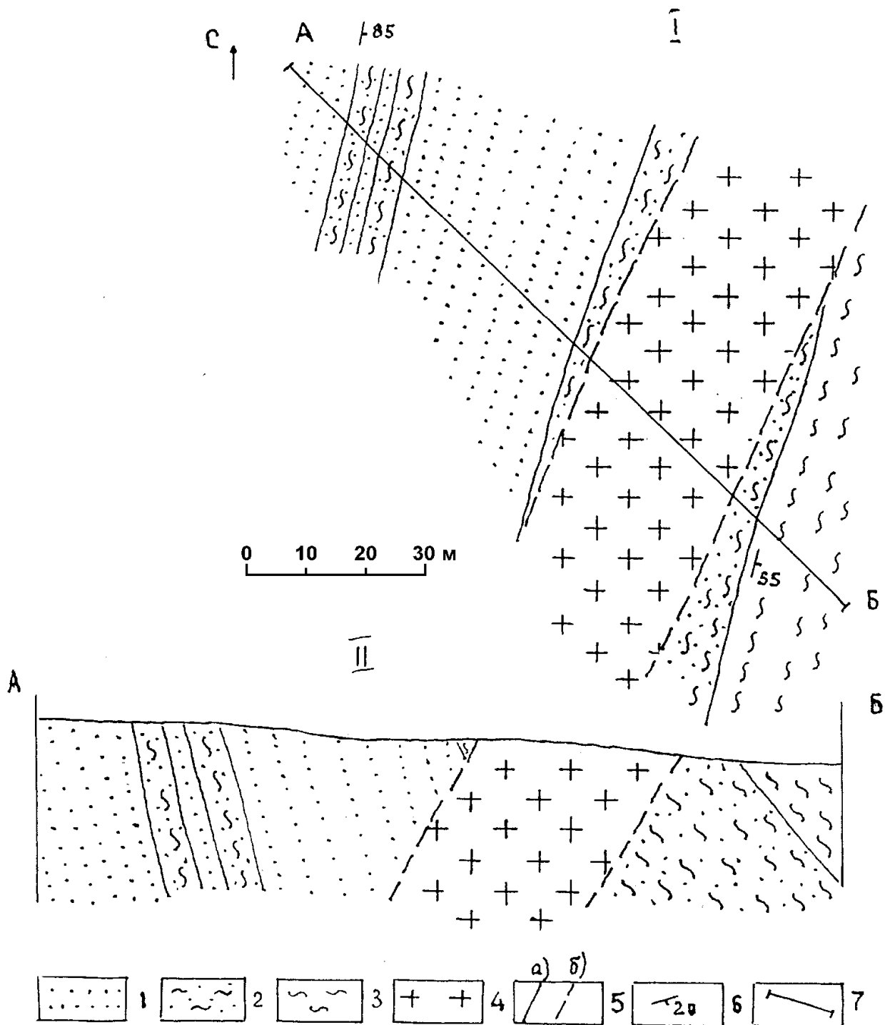
Рис. 8. Строение зоны контакта кизильской и березовской свит, из [3]
