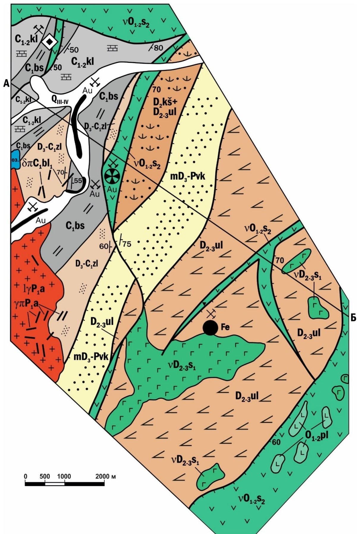
Рис. 3. Фрагмент геологической карты Атлянского полигона, по [3] с дополнениями. Условные обозначения см. приложение 7
