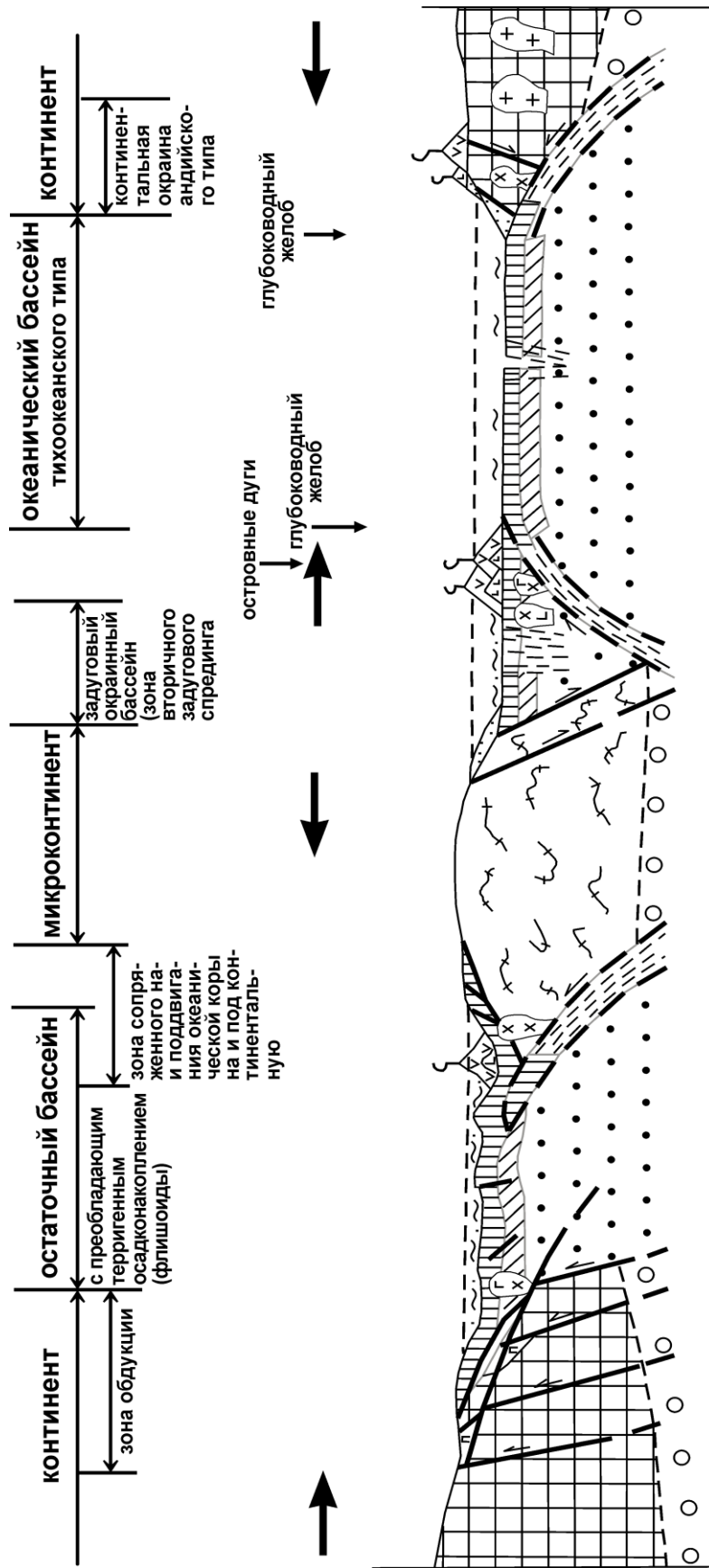
Рис. 13. Палеогеодинамические обстановки Палеоуральского океана в силуре – раннем карбоне, из [3] Условные обозначения см. на рис.унке 15
