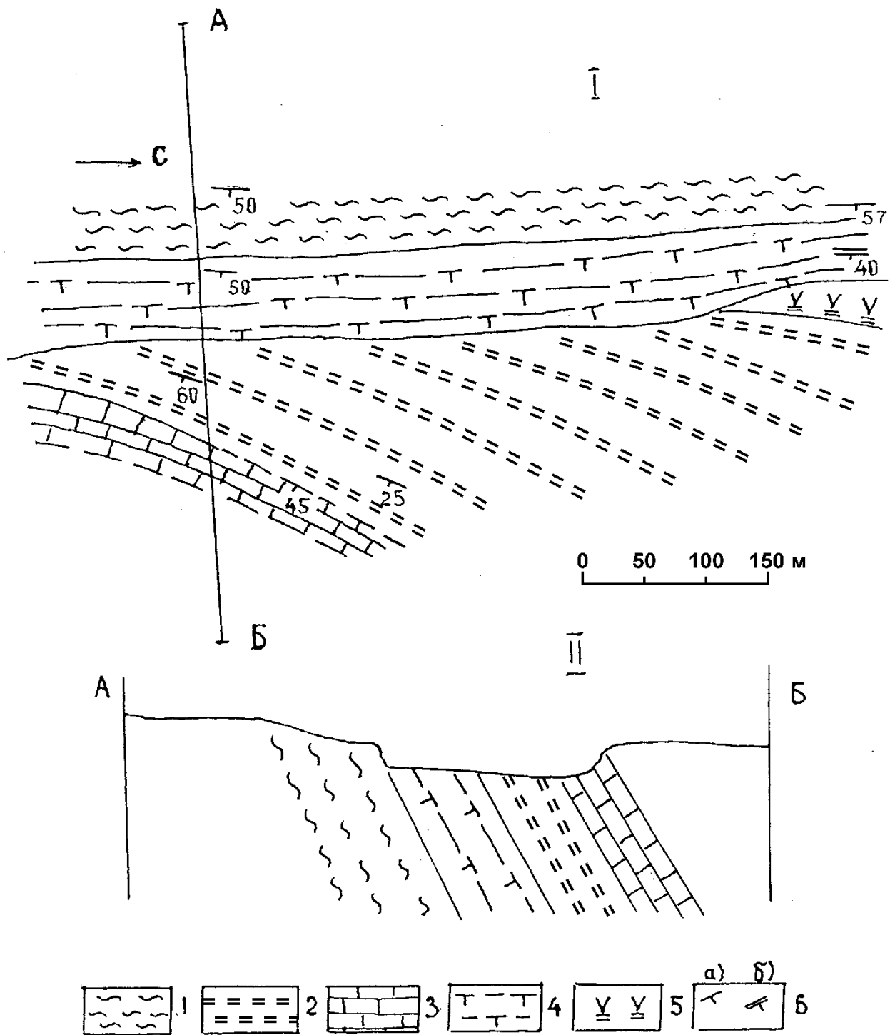
Рис. 9. Контакт уреньгинской и березовской свит с войкарско-кемпирсайским комплексом в районе карьера Сыростанского месторождения талька, из [3]
