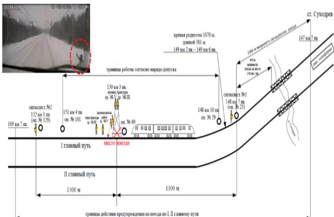
Рис. 1. Схема наезда подвижного состава на изолирующую съёмную вышку
