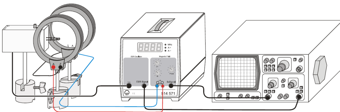
Рисунок 5. Экспериментальная установка для наблюдения спектров ЭПР радикала ДФПГ
