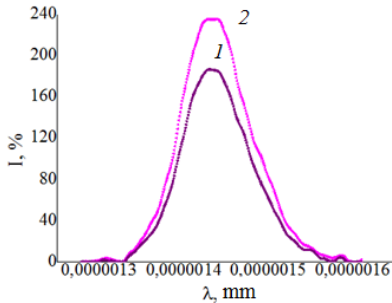
Рис. 2 Спектральная характеристика арсенид-галлиевого эпитаксиально излучающего диода 3Л129 при разных токах нагрузки: 1 – 100 мА; 2 – 50 мА
