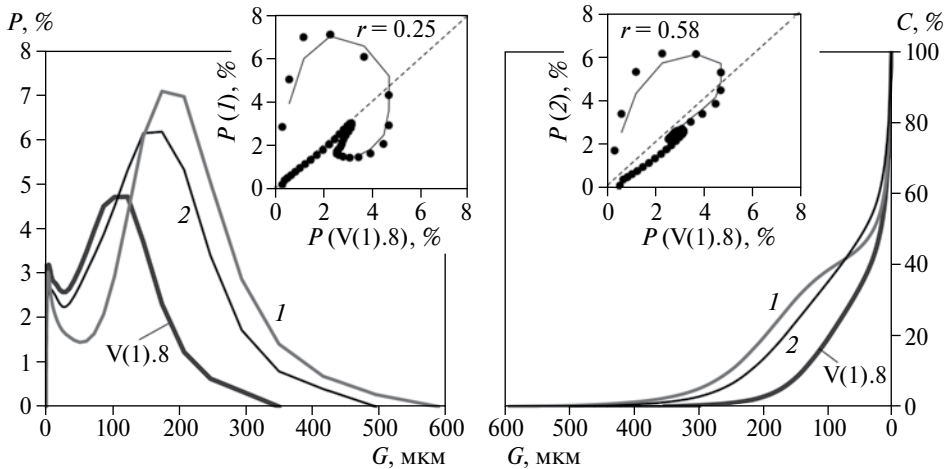
Рис. 3. Строение и состав аллювия V нпт (прибровочная часть, разрез V(1), см. рис. 1 и 2) долины р. Шура-Озень V(1).1, V(1).2 ... V(1).7 – фации (слои) аллювия террасы (в том числе V(1).3 и V(1).5 – гравийно-галечные русловые). На графиках показаны результаты гранулометрического анализа резко разнозернистых песчано-глинисто-алевритовых отложений, вскрываемых соответственно: V(1).8 – под аллювием V террасы (линзы (слои) ингрессионных глин (алевритов) Каспия гирканского времени?), 1 – в верхней части правого борта долины р. Шура-Озень под Малым Сарыкумом (образец 1, см. рис. 2) и 2 – на предположительно эрозионно-аккумулятивной (недатированной) террасе реки в Капчугайском ущелье; G – размерность ГМС, P – частоты встречаемости ГМС-элементов данной размерности, C – кумулятивные частоты ГМС-элементов, r – коэффициент линейной корреляции
