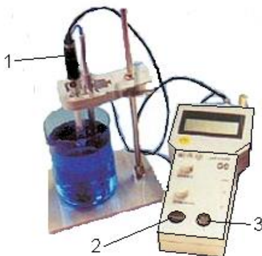
Рисунок 11 рН-метр рН-150
