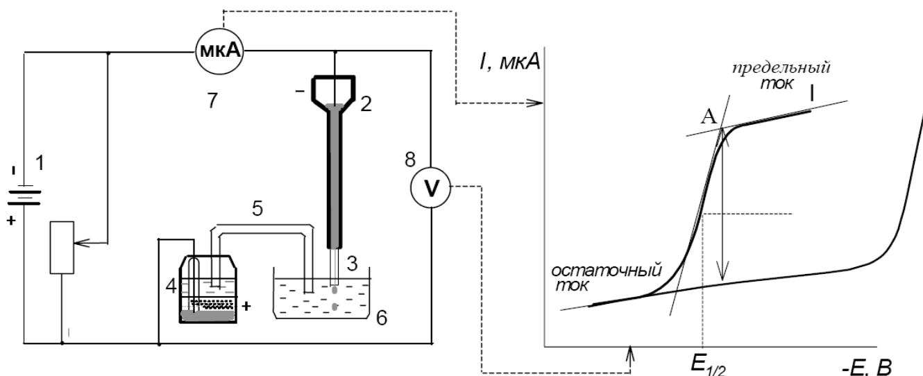
Рисунок 10 Схема полярографической установки (а): 1 – источник постоянного тока; 2 – резервуар с ртутью; 3 – капающий ртутный электрод (катод); 4 – насыщенный каломельный электрод (анод); 5 – солевой мостик; 6 – ячейка; 7 – микро-амперметр; 8 – вольтметр. Типичная полярограмма (б) депполяризатора (I) и фона (II).
