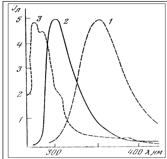
Рисунок 6. Спектры люминесценции аминокислот в нейтральном водном растворе при комнатной температуре. 1 – триптофан; 2 – тирозин; 3 – фениланин.
