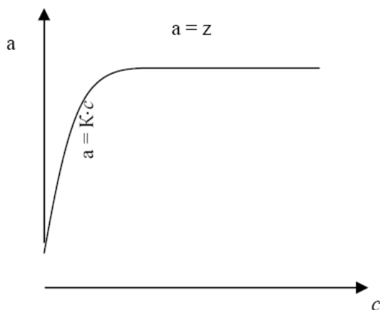
Рисунок 12 Изотерма адсорбции
