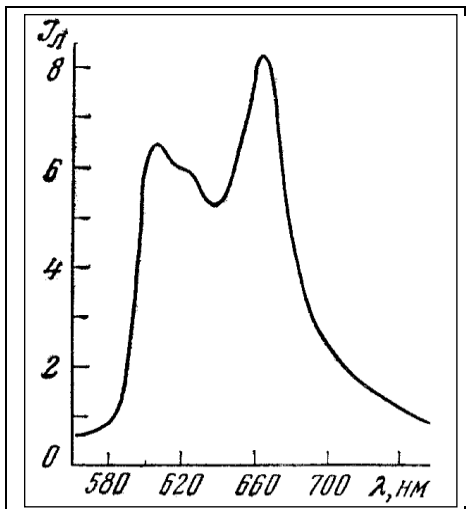
Рисунок 7. Спектр люминесценции гематопорфирина в эритроцитах, обработанных концентрированной кислотой. Длина волны возбуждения 436 нм.
