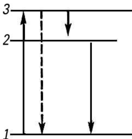
Рисунок 5. Схема квантовых переходов при элементарном процессе люминесценции: 1 — основной энергетический уровень; 2 — уровень излучения; 3 — уровень возбуждения. Переход 3—1, показанный пунктирной стрелкой, соответствует резонансной люминесценции, переход 2—1 — спонтанной люминесценции.
