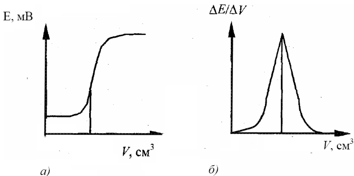
Рисунок 8 Кривые потенциметрического титрования: а) зависимость E от V; б) зависимость \Delta E/\Delta V от V
