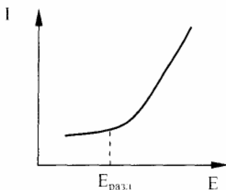
Рисунок 9 Кривая зависимости I = f(E)
