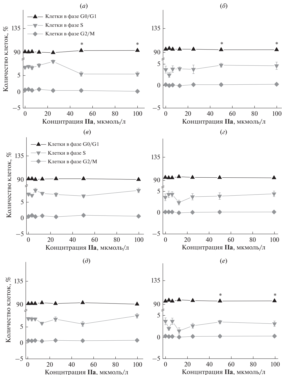
Рис. 5. Зависимость количества клеток в определенных фазах клеточного цикла от концентрации соединения (IIa), (IIc) и (IId) через 24 часа (a, в, д соответственно) и 48 часов инкубации (б, г, е соответственно). * – различия с интактными клетками (на графике – концентрация 0 мкмоль/л) статистически достоверное при p < 0.05 (тест Манн–Уитни).
