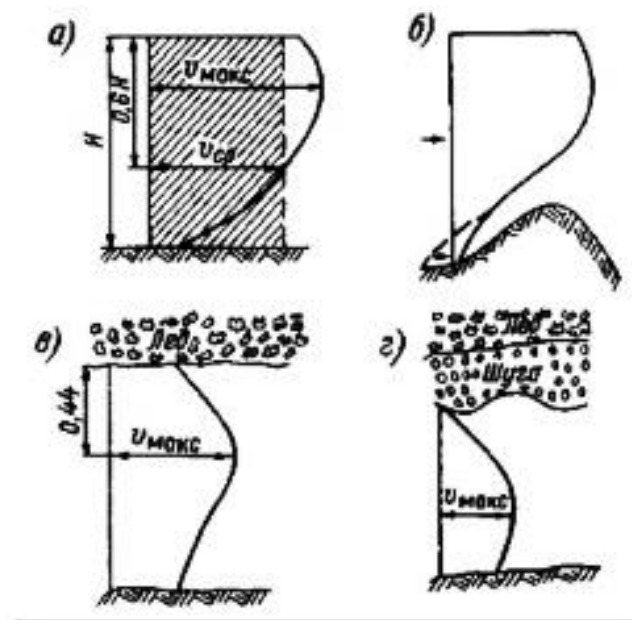
Рис. 1. 2. Распределение скоростей в речном потоке: а — открытое русло, б — перед препятствием, в — ледяной покров, г — скопление шуги
