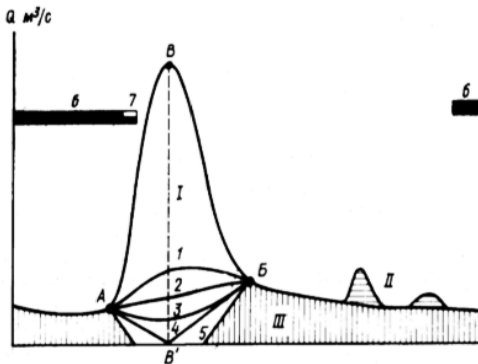
Рис. 1.4. Расчленение гидрографа реки (объяснения в тексте)
