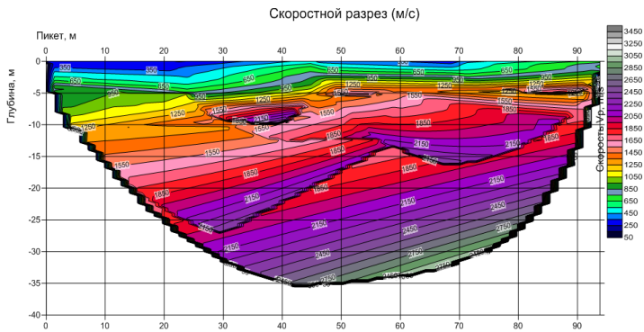
Рисунок 2 – Скоростной разрез продольных волн, профиль ПР01
