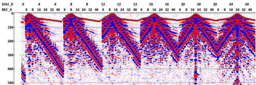
Рисунок 1– Сейсмограммы продольных волн
