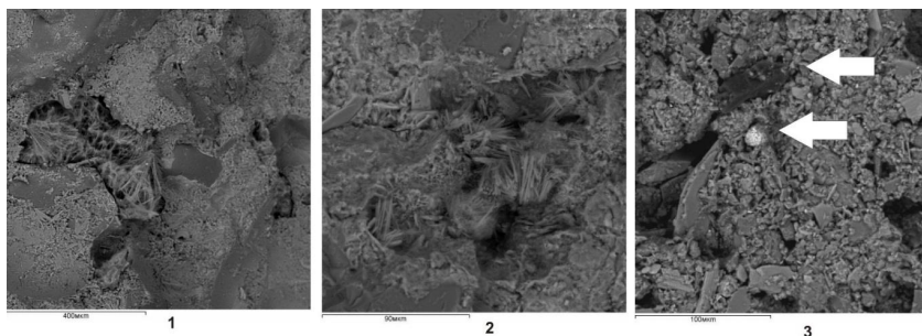
Рисунок 1 – Строение цементного камня изученной плитки:
