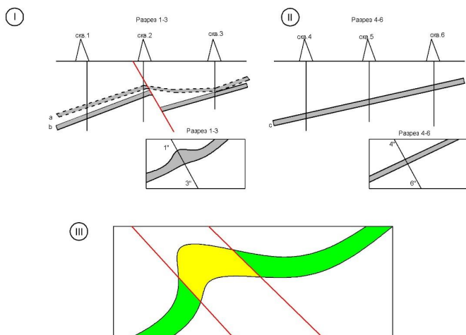
Рисунок 1 – Схематическая иллюстрация различных типов залегания пласта Одинокого на месторождении «Фандюшкинское поле»
