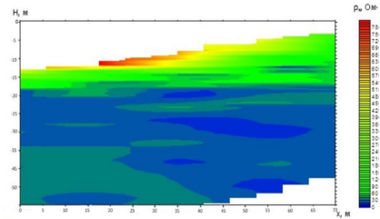
Рисунок 2 – Зависимость удельного сопротивления от глубины на ПК-108
