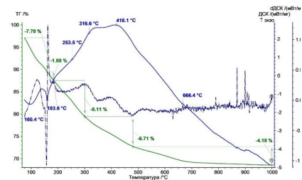
Рисунок 2 – Результаты СТА смеси Са-стильбита и смектита (75:25)
