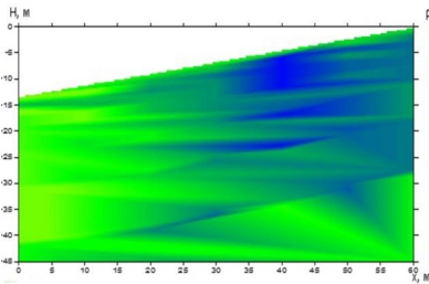
Рисунок 1 – Зависимость удельного сопротивления от глубины на ПК-54
