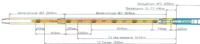
Рисунок 1 – Структурная схема забойной телеметрической системы ЗТС-48
