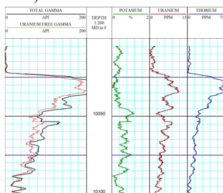
Рисунок 2 – Результаты данных спектрального гамма-каротажа
