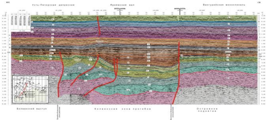
Рисунок 1 – Составной временной разрез по сейсмическим профилям
