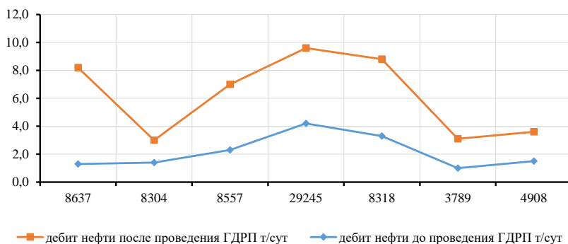
Рисунок 1 – Изменение дебита нефти
