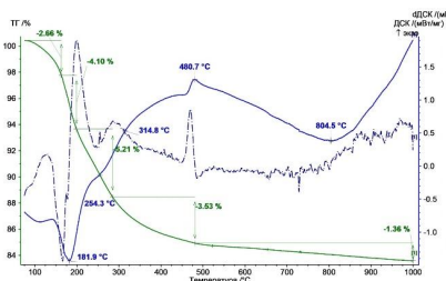
Рисунок 1 – Результаты СТА Са-стильбита автора
