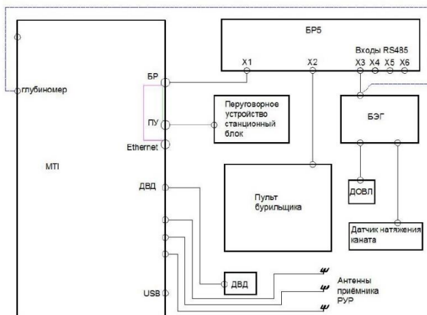
Рисунок 2 – Структурная схема наземной системы МТП
