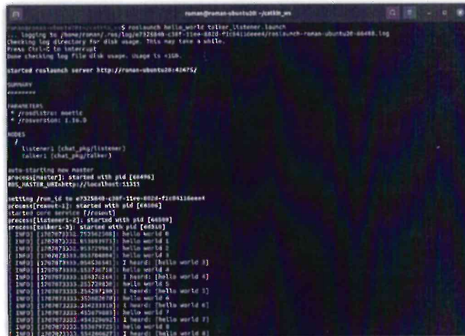
Рис. 3.6: Вывод при запуске файла talker_listener.launch.
