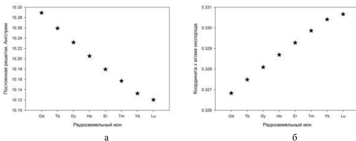
Рисунок 1. Зависимость постоянной решетки (а) и координаты x кислорода (б) от редкоземельного иона в структуре R_2Ti_2O_7 (R = Gd – Lu)
