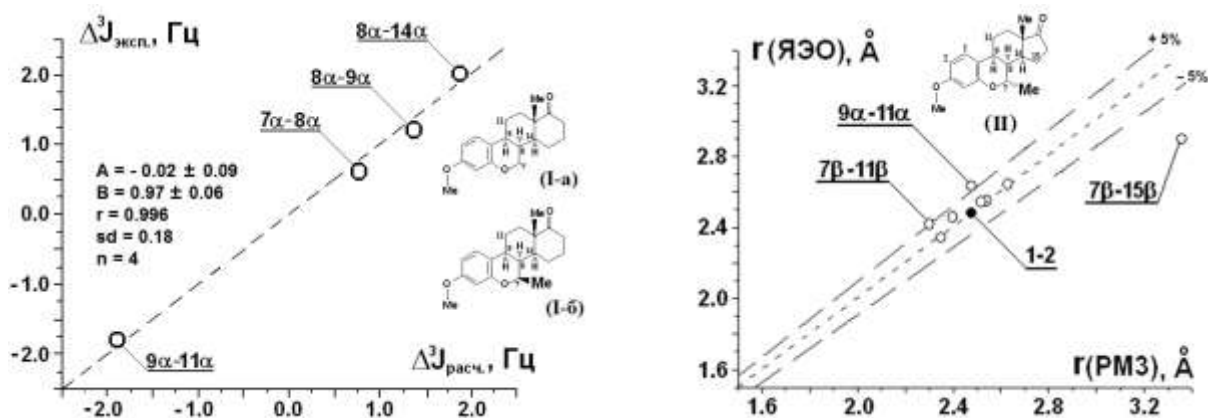
Рис. 1. Примеры использования {}^3J (слева) и r (справа) для изучения строения и динамики стероидов (I) и (II), соответственно. \Delta{}^3J = {}^3J^{(I-b)} - {}^3J^{(I-a)} ; ● – эталонное расстояние 2.48 Å.
