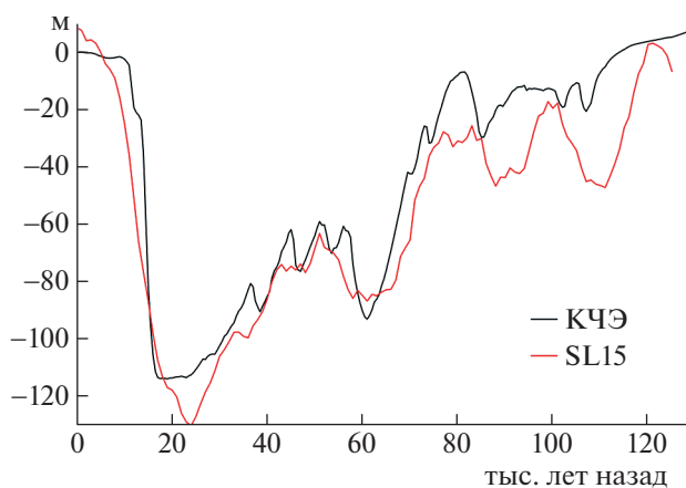
Рис. 1. Изменения глобального уровня океана в контрольном численном эксперименте (черная кривая) с моделью ледовых щитов в сравнении с данными палеореконов [14] (красная кривая).
