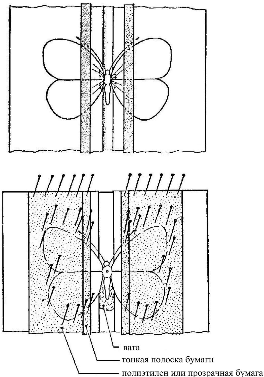
Рис. 15. Схема расправления бабочки (по Koch, 1984)
