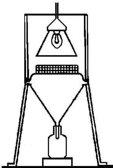
Рис. 7. Конструкция эклектора (по Гилярову, 1975 б).
