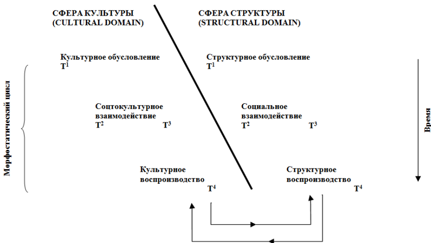
Рис. 4. Различиях морфогенеза и морфостазиса (воспроизводство)
