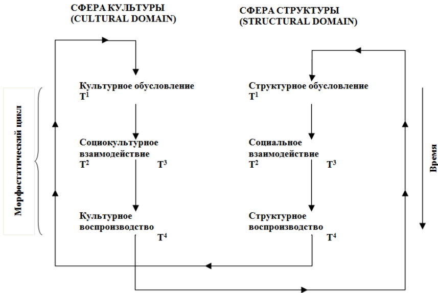
Рис. 3. Различиях морфогенеза и морфостазиса (выработка)
