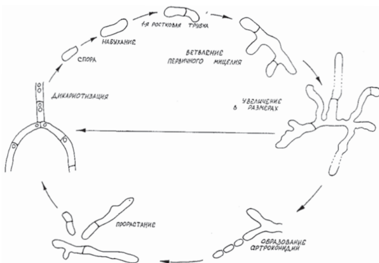
Рис.2. Жизненный цикл видов рода Trametes .
