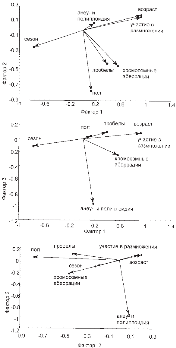
Рис.1. Факторный анализ изменчивости хромосомных нарушений у рыжей полевки из Шигаево.
