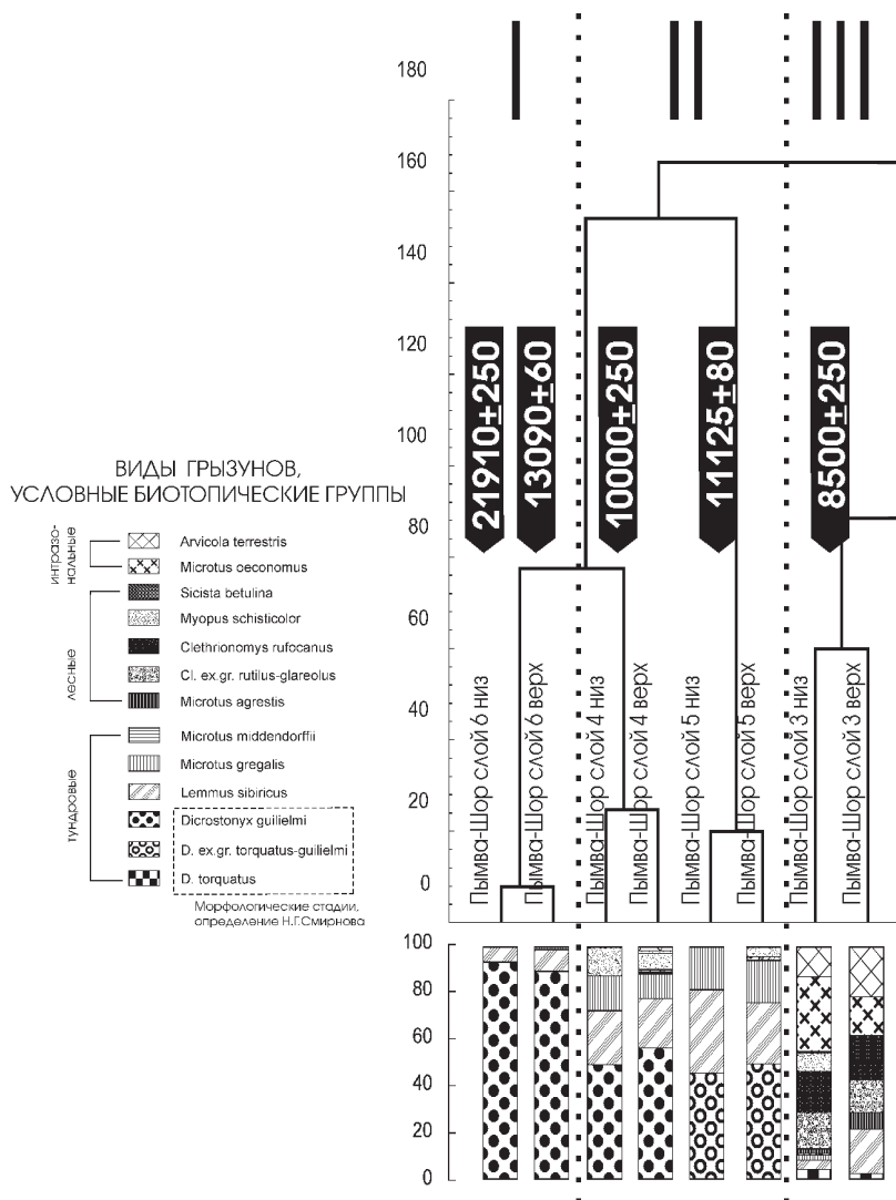
Рисунок. Основные типы фаун грызунов позднечетвертичных местонахождений Приуральской Субарктики.
