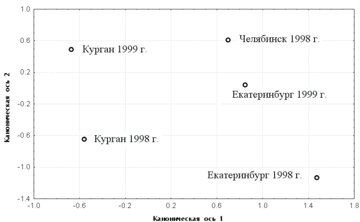
Рисунок. Дискриминантный анализ трофических показателей самок разных микропопуляций зауральской популяции непарного шелкопряда.
