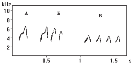
Рис. 2. Характеристики частотной модуляции (сонограммы) звукового предупреждающего об опасности сигнала краснощекого суслика (Б, В — серии криков).
