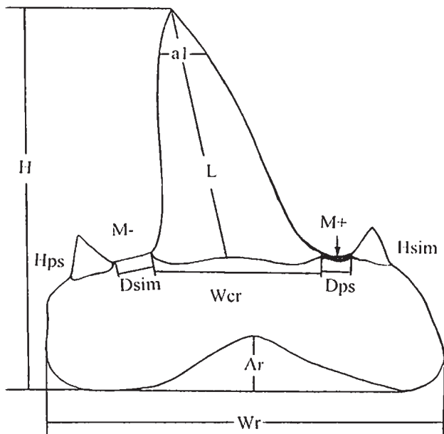
Рис.2. Схема промеров: H — высота зуба; L — длина коронки; Wcr — ширина основания коронки; Wr — ширина корня; Ar — высота арки корня; Hsim , Hps — высота бокового зубца с симфизарной и противосимфизарной сторон; Dsim , Dps — промежуток между главной и боковыми вершинами; M , M+ — наличие или отсутствие эмалевого мостика между главной и боковыми вершинами.
