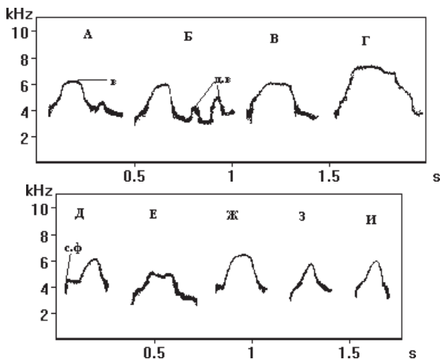
Рис. 3. Сонограммы звукового предупреждающего об опасности сигнала сусликов из популяций гибридной зоны (в — вершина характеристики частотной модуляции, д.в — дополнительная вершина характеристики частотной модуляции, с.ф. — ступенчатая флуктуация частотной модуляции сигнала).
