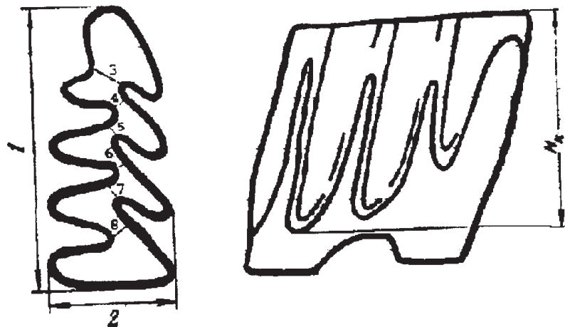
Рис. 1. Схема промеров: 1 — длина зуба, 2 — ширина зуба, 3—8 ширина слияний дентиновых полей, H_k — высота коронки.
