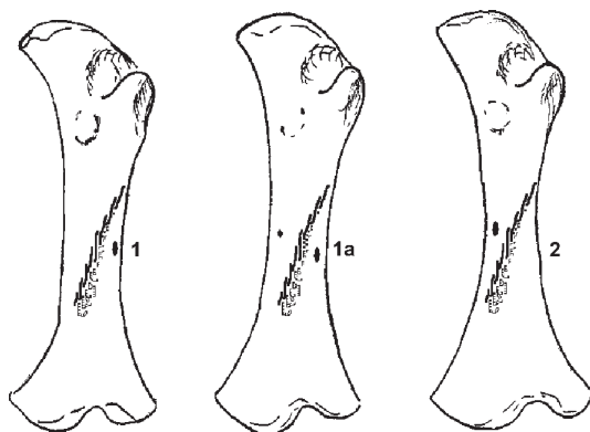
Рис. 3. Расположение питательных отверстий на бедренной кости ( femur, dexter, juvenis ). Вентральный вид.
