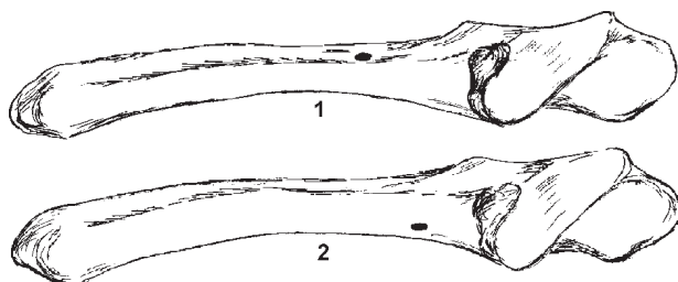
Рис. 2. Расположение питательного отверстия на локтевой кости ( ulna, dexter, juvenis ). Дорзальный вид.
