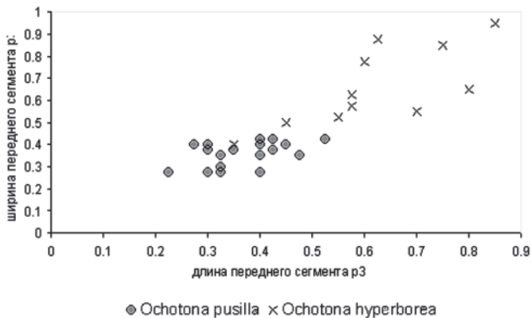
Рис. 2. Размерные характеристики переднего сегмента р3 рецентных пищух.
