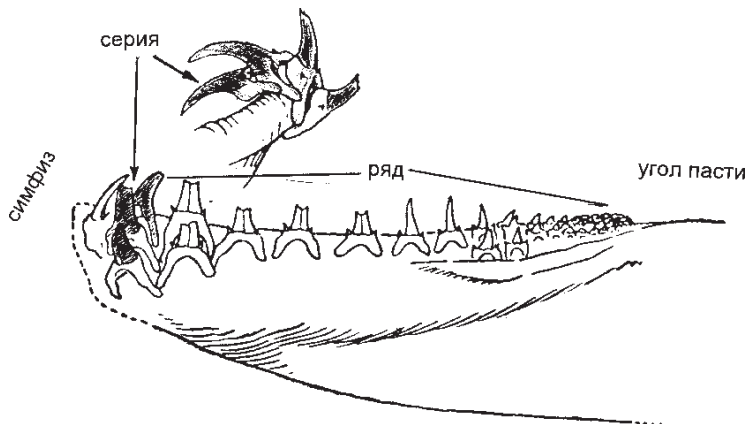
Рис. 3. Строение челюсти ламноидной акулы.
