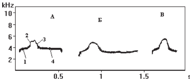
Рис. 1. Характеристики частотной модуляции (сонограммы) звукового предупреждающего об опасности сигнала рыжеватого суслика (1-4 — фазы частотной модуляции сигнала).
