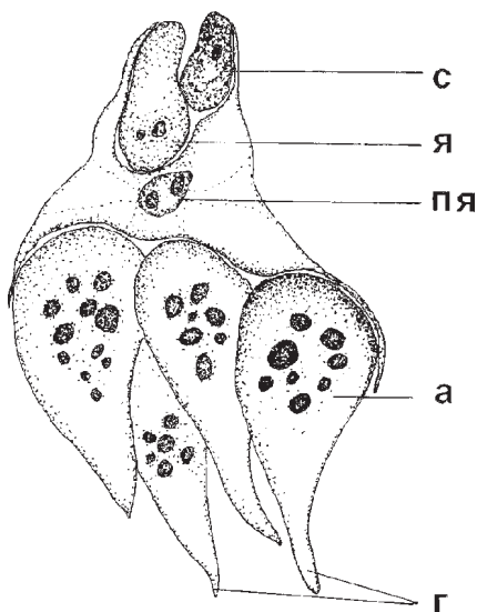
Рис. 1. Зародышевый мешок P. alpigena с гаусториальными выростами антипод ( г ). Обозначения: а — антиподы, п я — полярные ядра, с — синергида, я — яйцеклетка.
