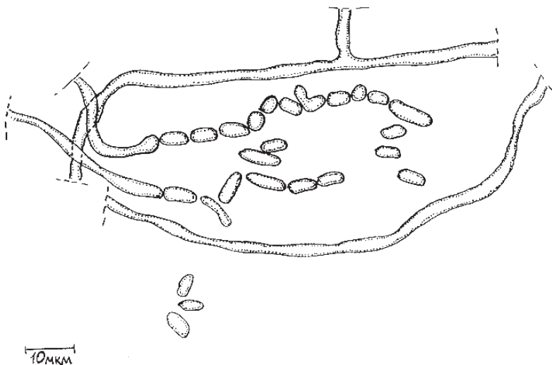
Рис. 1. Образование артроконидий Trametes hirsuta (x400).
