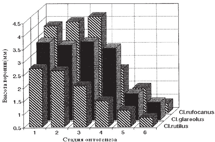
Рис. 2. Изменение размерных характеристик зубов в зависимости от стадии онтогенеза у лесных полевок: А — среднее значение длины зуба, Б — среднее значение высоты коронки.
