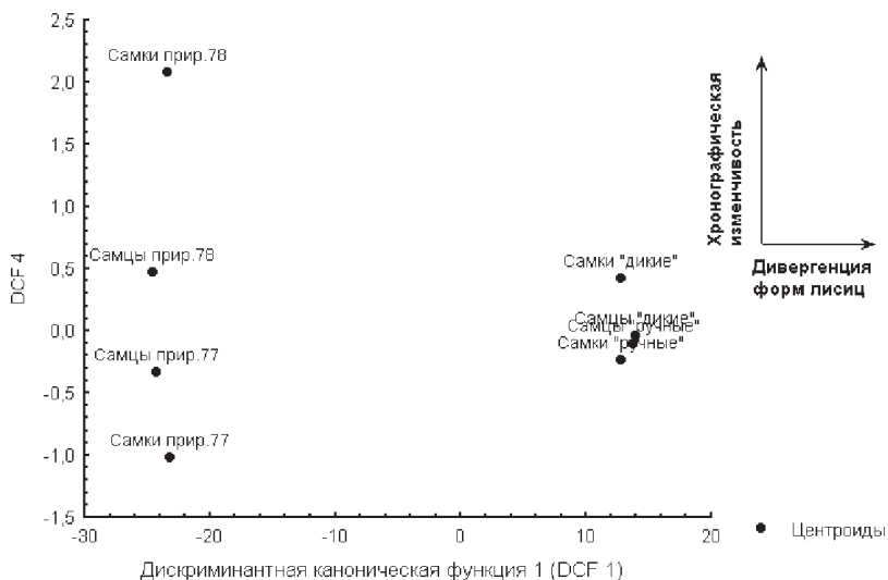
Рис.3. Дискриминантный анализ формы и размеров черепа сравниваемых групп лисиц с учетом хронографической изменчивости природной популяции.
