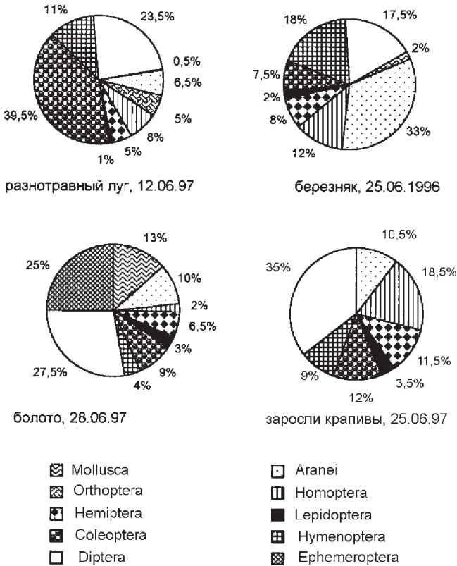
Рис. 1. Соотношение основных групп беспозвоночных в травостое разнотипных сообществ.
