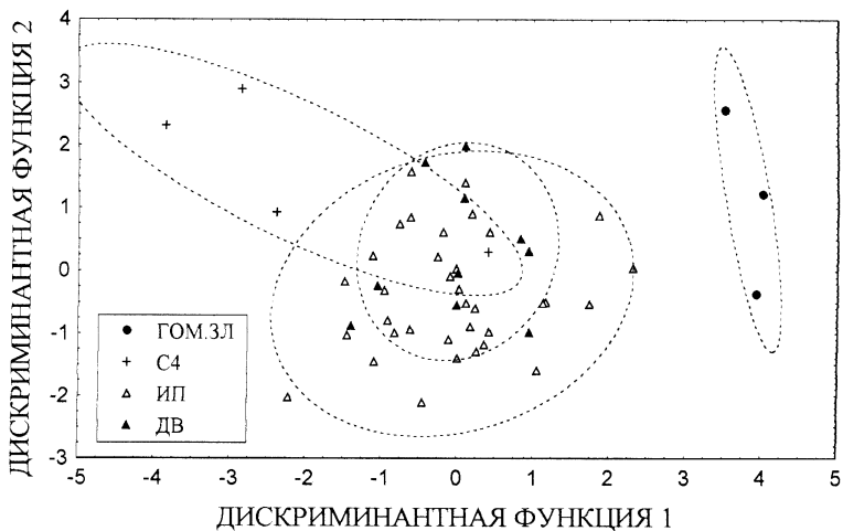
Рис.3. Дискриминантный анализ групп растений с разным типом строения мезофилла листа.
