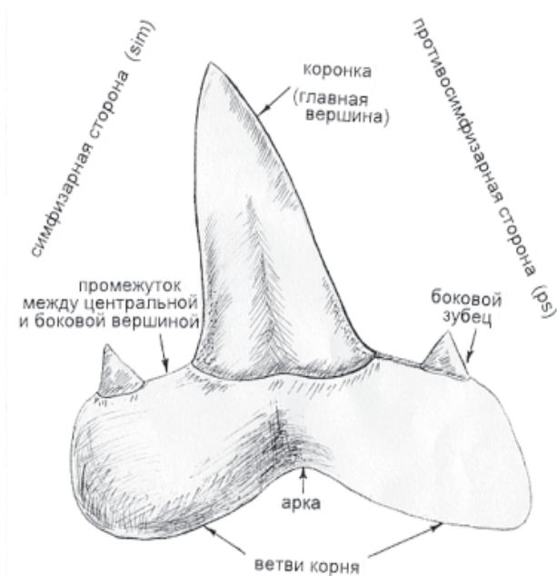
Рис.1. Строение зуба ламноидной акулы.
