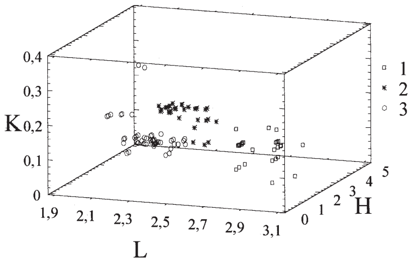
Рис. 3. Соотношение длины зуба ( L , мм), высоты коронки ( H , мм) и индекса отношения ширины дентинового слияния призм параконидного отдела к ширине жевательной поверхности ( K ) у современных полевок рода Clethrionomys : 1 — Cl. rufocanus ; 2 — Cl. glareolus ; 3 — Cl. rutilus .
