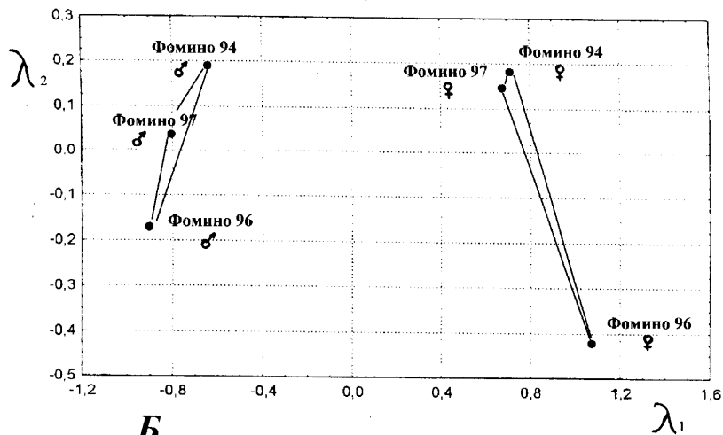
Рис. 4. Соотношение хронографических, хорологических и половых различий (дискриминантный анализ). А — Coenonympha glycerion ; Б — Coenonympha arcania .
