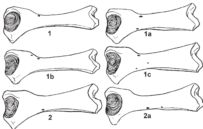
Рис. 4. Расположение питательных отверстий на плечевой кости ( humerus, sinister, juvenis ). Вентральный вид.
