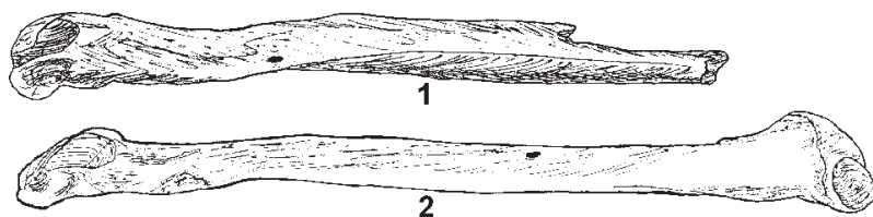
Рис. 1. Расположение питательного отверстия на малой берцовой кости ( fibula, sinister, adultus ). Дорзальный вид.
