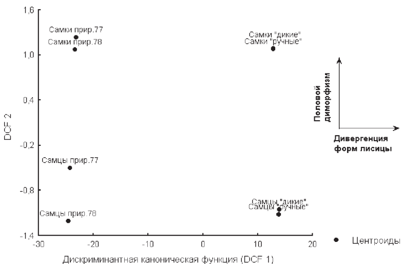
Рис. 1. Дискриминантный анализ формы и размеров черепа сравниваемых групп лисиц: анализ проявления полового диморфизма.
