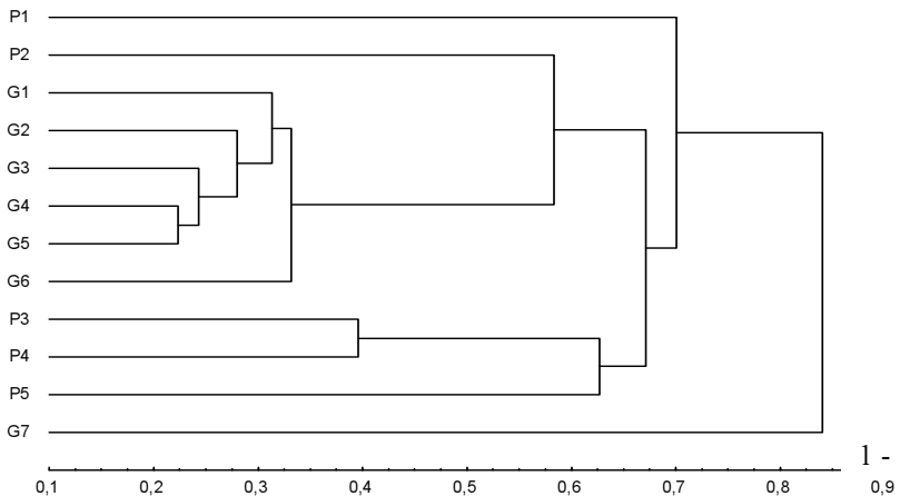
Рис.2. Дендрограмма сходства глазчатых пятен крылового рисунка самок Coenonympha glycerion . (Пятна рисунка переднего крыла обозначены буквами P, пятна заднего крыла — буквами G).
