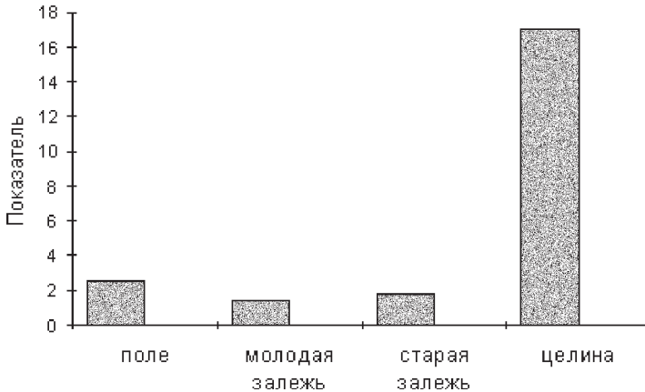
Рис.2. Общая устойчивость сообществ мелких млекопитающих исследованных местообитаний.
