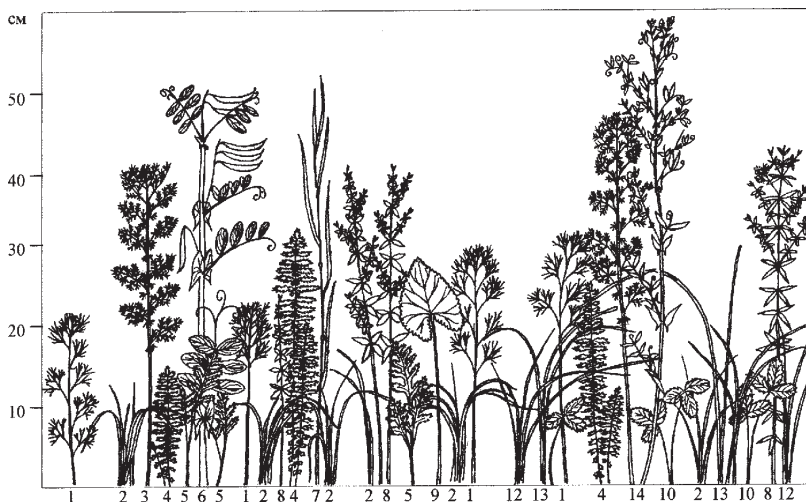
Рис. 5. Разнотравно-североподмаренниково-шелковистопольная луговая степь (вертикальная проекция, июль 1999г.). 1 — Artemisia sericea , 2 — Carex supina , 3 — Artemisia pontica , 4 — Filipendula vulgaris , 5 — Artemisia latifolia , 6 — Lathyrus pisiformis , 7 — Elytrigia lolioides , 8 — Galium boreale , 9 — Phlomidoides tuberosa , 10 — Fragaria viridis , 11 — Phleum phleoides , 12 — Carex praecox , 13 — Poa angustifolia , 14 — Lathyrus pratensis .
