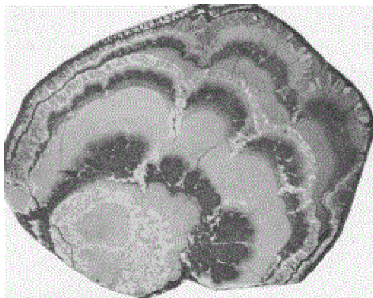
Рис. 5. Колломорфная текстура агрегата псиломелана (светло-серое), с трещинками усыхания) и халцедона (черное). Структура агрегата псиломелана и халцедона гелевая. Для пиролюзита (белое) характерны волокнистая метаколлоидная структура и колломорфная метаколлоидная текстура. Полированный штуф.
