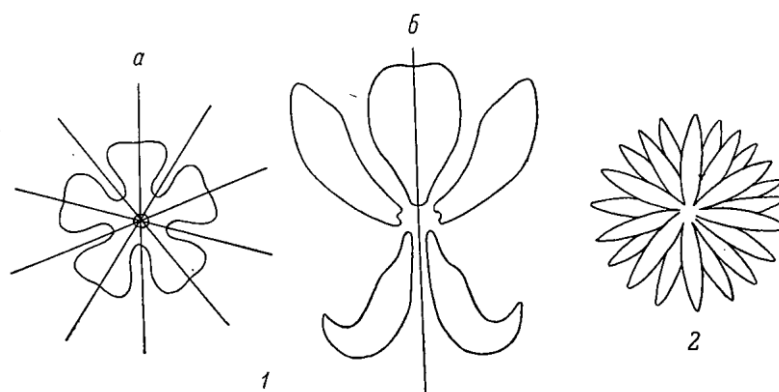
Рисунок 2. Различные формы симметрии цветка 1 – цветки симметричные: a – актиноморфный, б – зигоморфный; 2 – цветок несимметричный.
