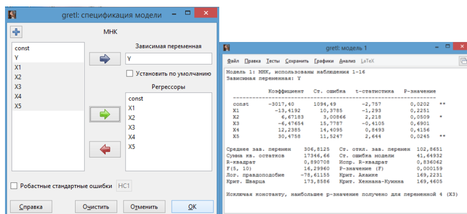
Рис. 1.1. МНК-оценки исходной регрессии
