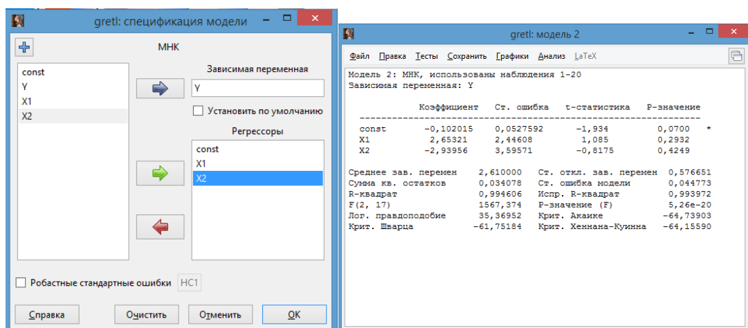
Рис. 2.1. Построение линейной модели регрессии с двумя факторами
