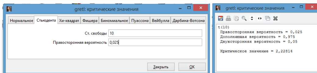
Рис. 1.3. Окно Инструмента «Критические значения» (Стьюдента)
