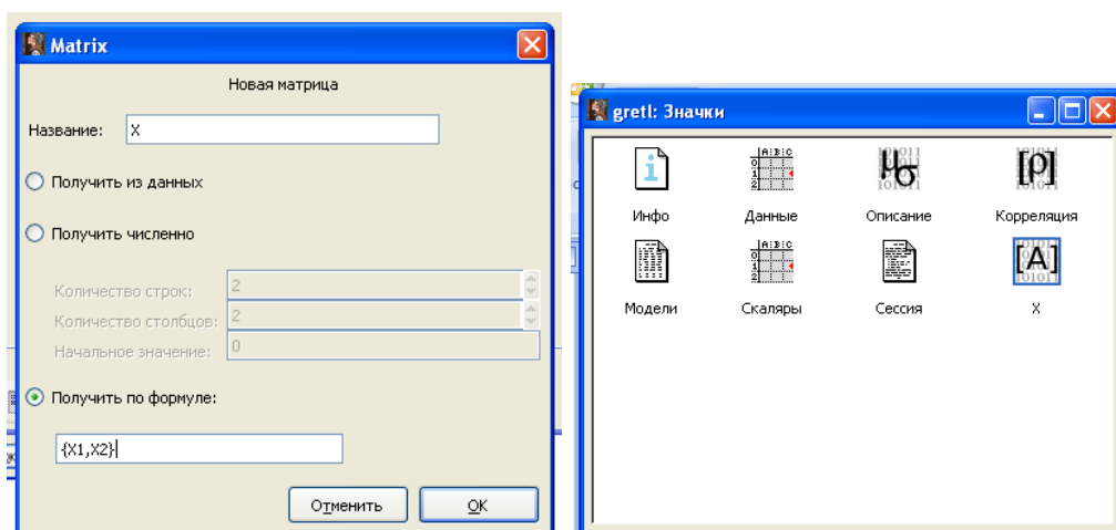
Рис. 1.10. Окно добавления матрицы регрессоров
