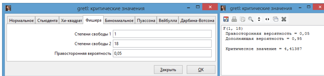
Рис. 1.17. Окно Инструмента «Критические значения» (Фишера)
