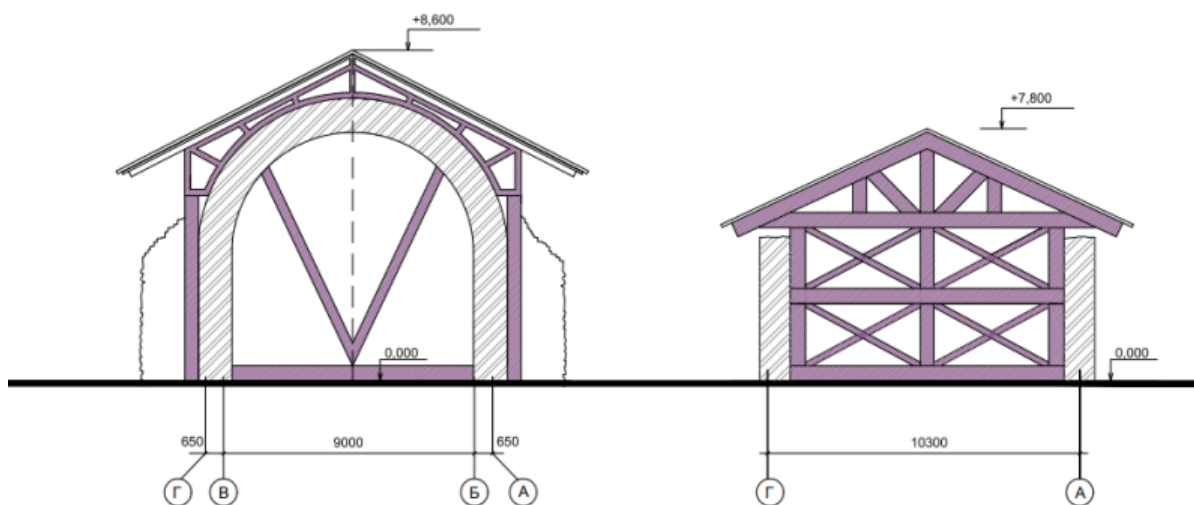
Рис.6. Схема устройства стропильной системы основного здания
