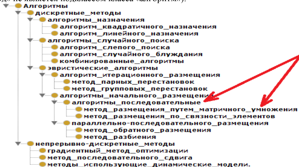
Рис.1. Пример типовой ошибки проектирования онтологии
