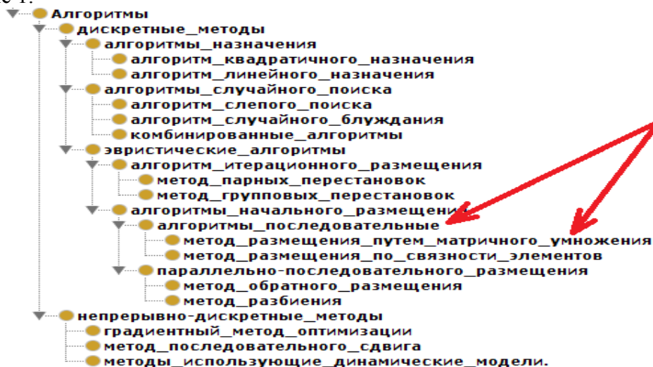
Рис. 1. Пример типовой ошибки проектирования онтологии
