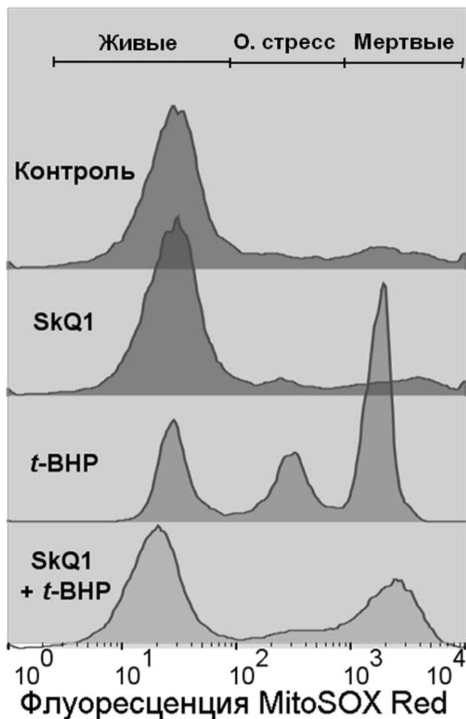
Рис. 1. Окислительный стресс в клетках D. magnusii . Антиоксидантное действие SkQ1.
