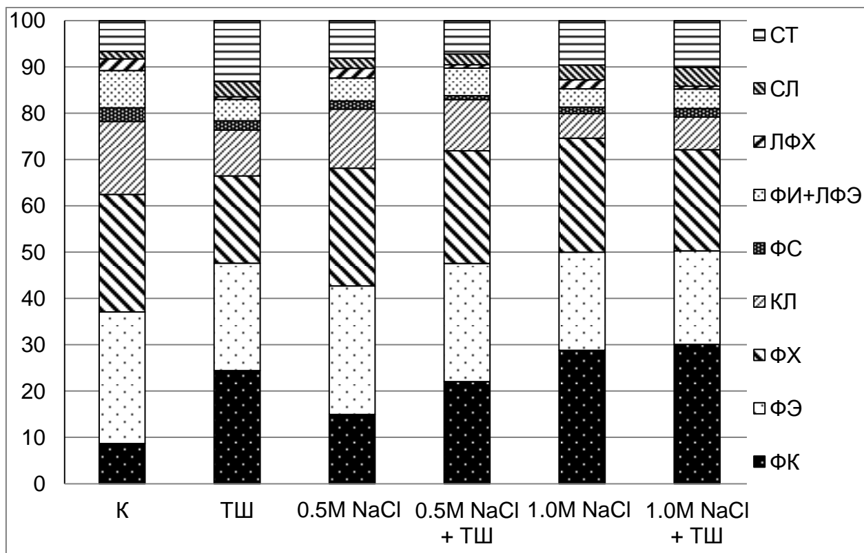
Рисунок 2. Состав мембранных липидов мицелиального гриба A. niger в условиях комбинированного действия теплового и осмотического шоков (% от суммы)
