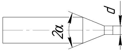
Рис. 5. Конус заточки
