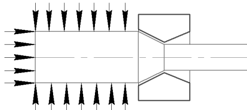
Рис. 2. Обычный способ гидропрессования
