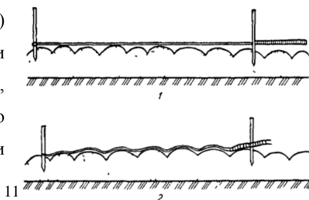
Рис.2. Измерение гребнистости
