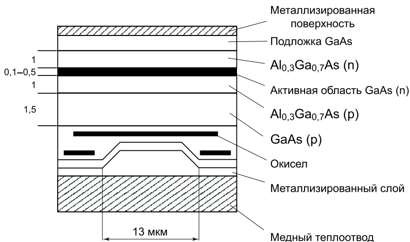
Рис. 10. Приблизительная реализация лазерного диода \text{Al}_{0,3}\text{Ga}_{0,7}\text{As} (p) – GaAs (p) и GaAs (n) – \text{Al}_{0,3}\text{Ga}_{0,7}\text{As} (n), активная область – слой из GaAs (n) [4]
