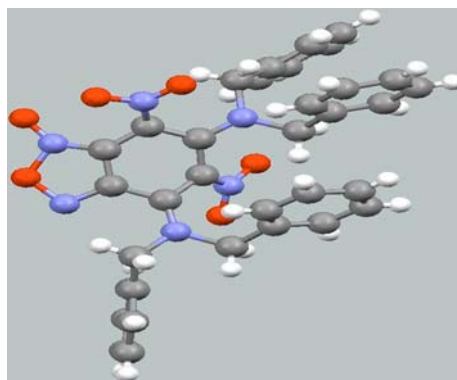
Рис. 9. Геометрия продукта 4 в кристалле
