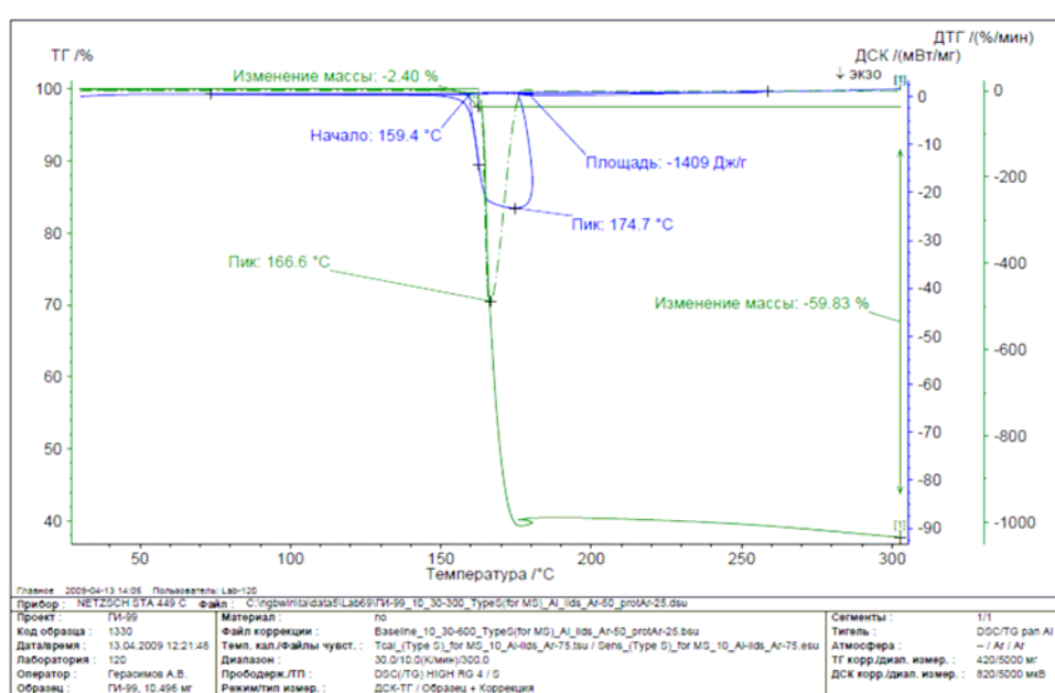
Рис. 6. Дериватограмма продукта 3
