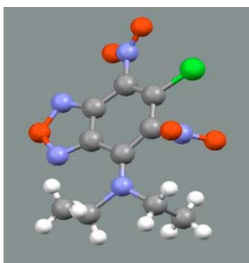
Рис. 15. Геометрия продукта 7 в кристалле по данным РСА
