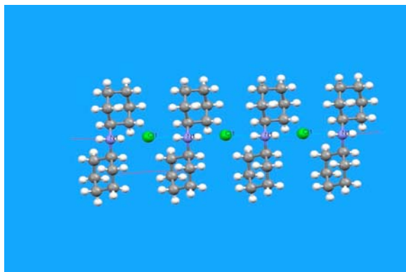
Рис. 10. Геометрия дициклогексиламмонийхлорида
