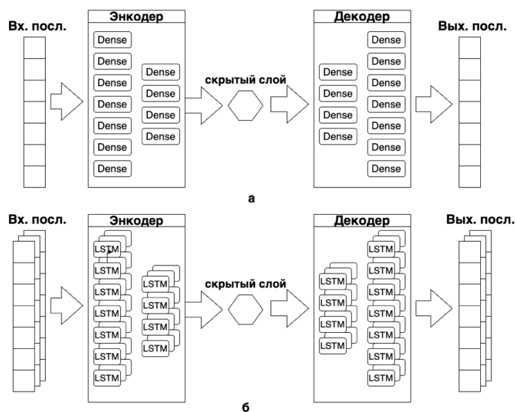
Рис. 1. Структура автоэнкодера
