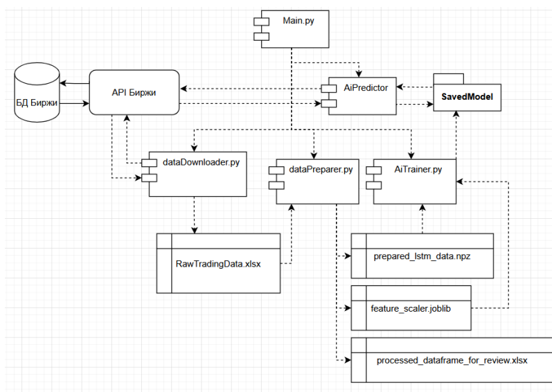
Рис. 4. Диаграмма компонентов
