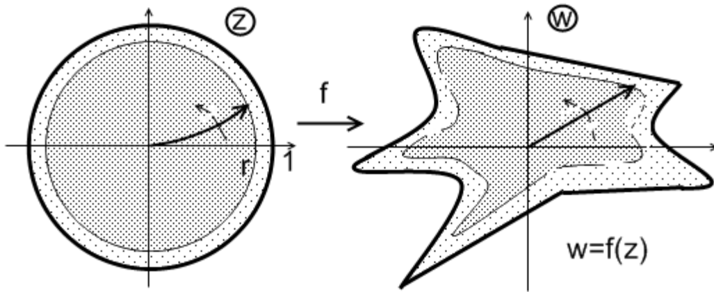
Рис. 13: Отображение на звездообразную область
