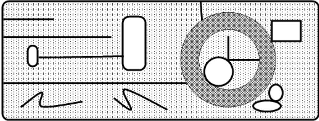
Рис. 18: Определение максимального модуля
