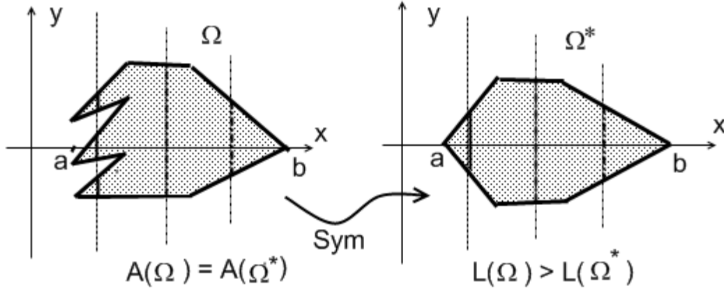
Рис. 15: Симметризация относительно прямой
