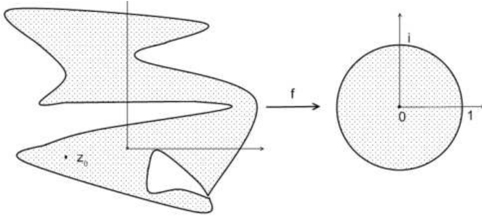
Рис. 3: К теореме Римана
