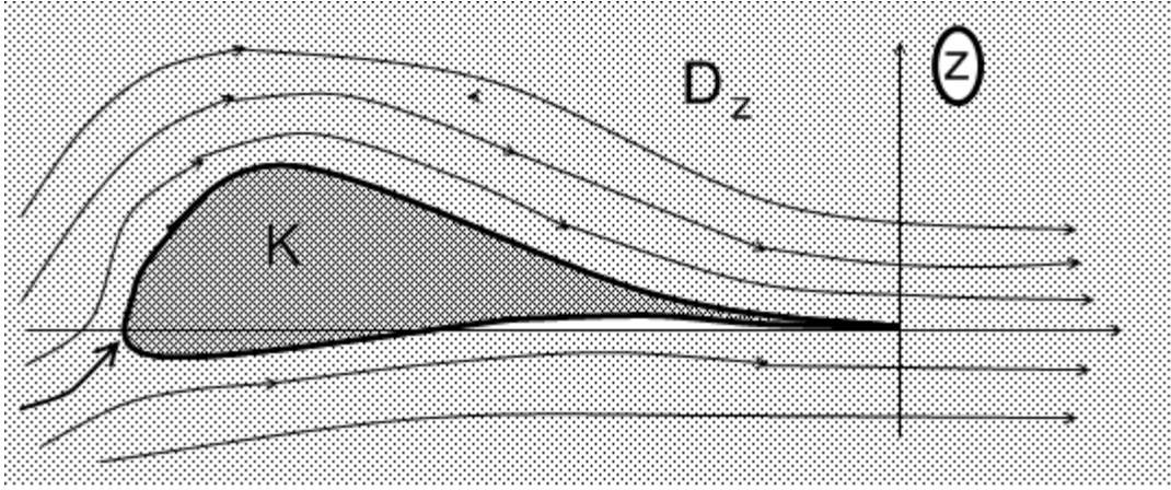
Рис. 16: Обтекание крыла K
