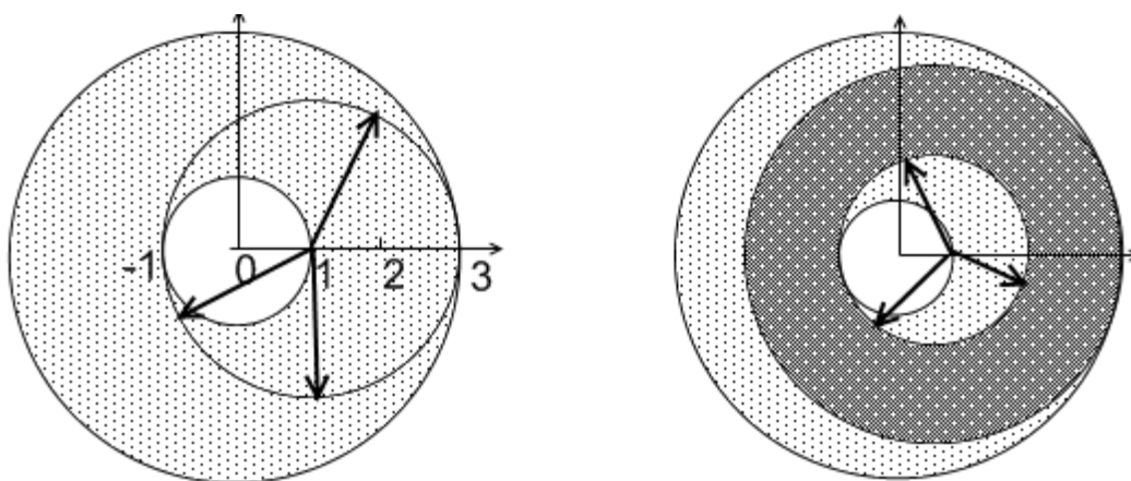
Рис. 19: Центр вложенного кольца – граничная точка большого кольца
