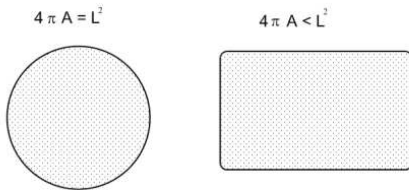
Рис. 9: Сравнение площади с длиной границы
