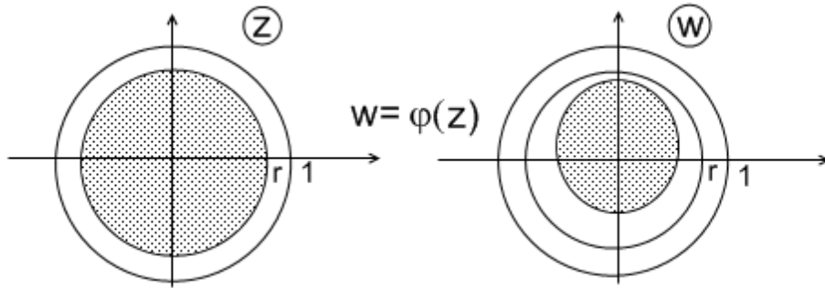
Рис. 7: К лемме Шварца
