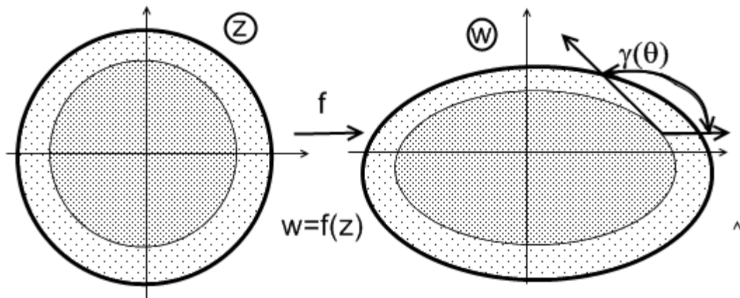
Рис. 14: Отображение на выпуклую область
