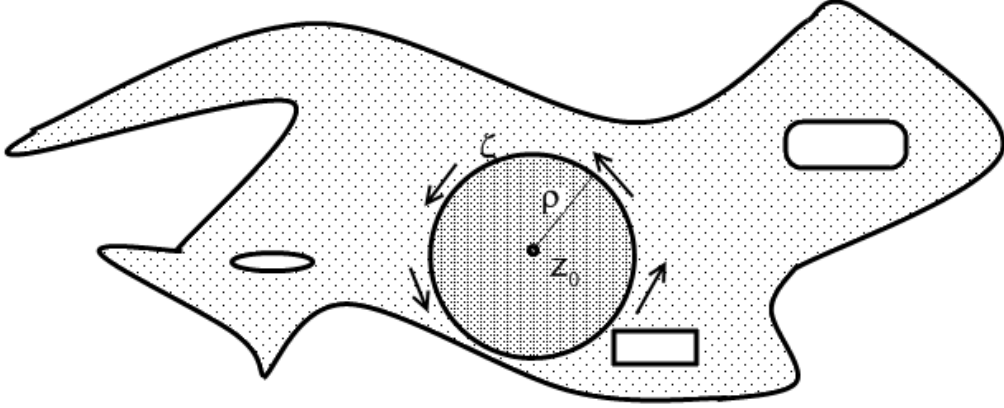
Рис. 2: К интегральной формуле Коши
