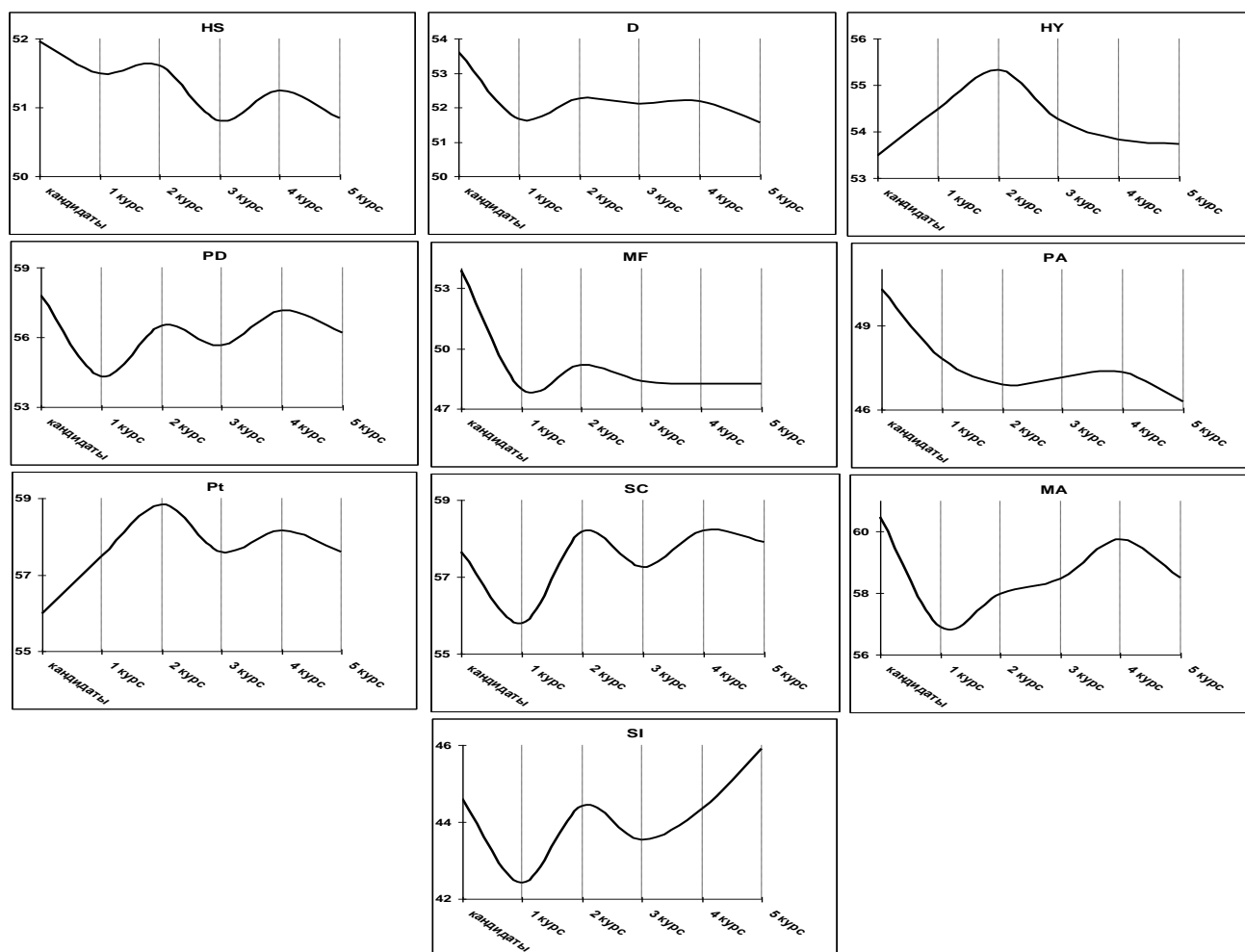
Рис. 1. Динамика шкал профиля личности курсантов в период обучения
