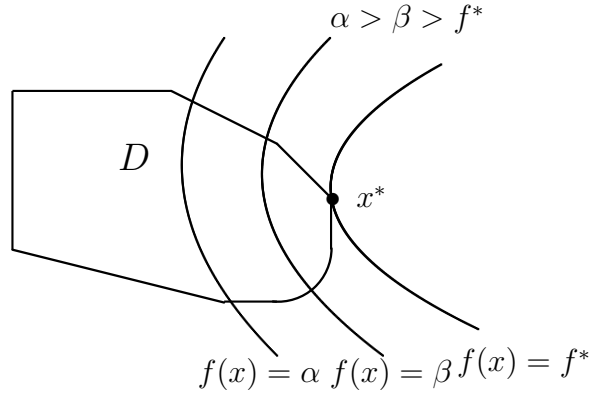
Рис. 1.1: Задача оптимизации при n = 2 , D^*(f) = \{x^*\} .
