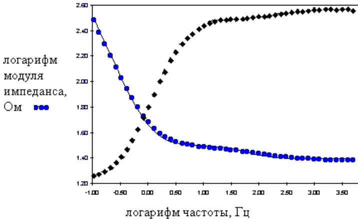
Рис. 4. Диаграмма Бодэ исследуемой системы
