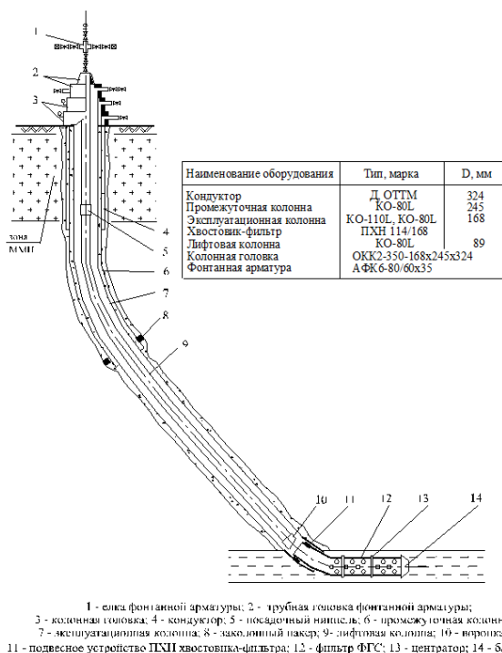
Рисунок 1.1. Принципиальная компоновка лифтовой колонны газоконденсатной наклонно-направленной скважины с горизонтальным окончанием ствола
