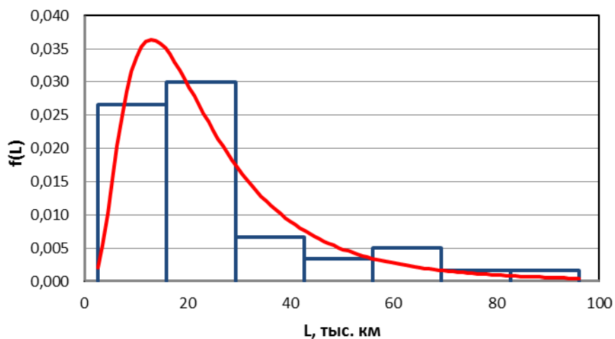
Рис. 2. Распределение наработок на отказ ремней поликлиновых БРК-1220
