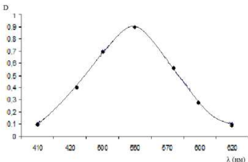
Рисунок 3 – Зависимость оптической плотности от длины волны
