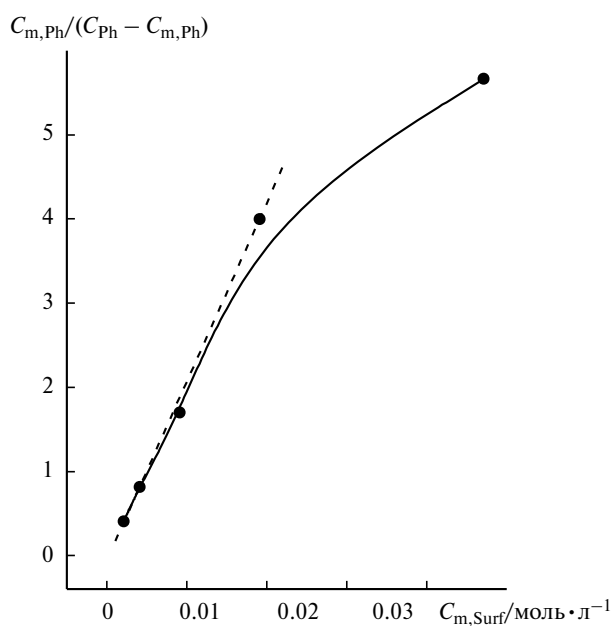
Рис. 3. Зависимость соотношения мольных концентраций фосфата 7 в мицеллярной и водной фазах от концентрации КПАВ 3 в составе мицелл.
