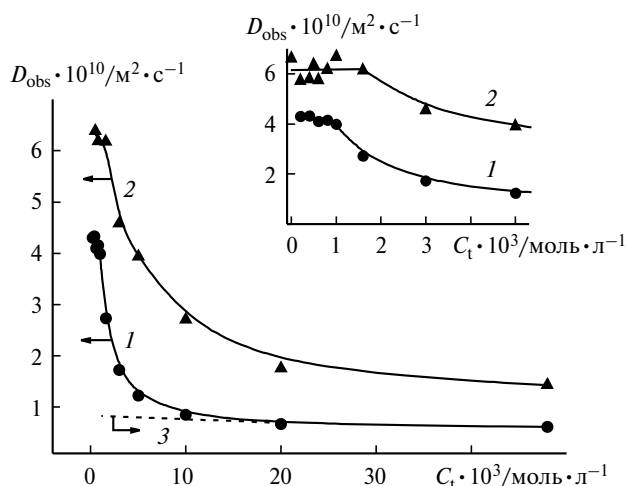
Рис. 1. Зависимость наблюдаемого коэффициента самодиффузии КПАВ 3 ( 1 ) и фосфата 7 ( 2 ) от концентрации ПАВ при 30 °С, C_T = 10^{-3} моль \cdot л ^{-1} ; касательная к кривой 1 при высоких концентрациях ПАВ ( 3 ). На вставке — зависимости 1 и 2 в области низких концентраций ПАВ.
