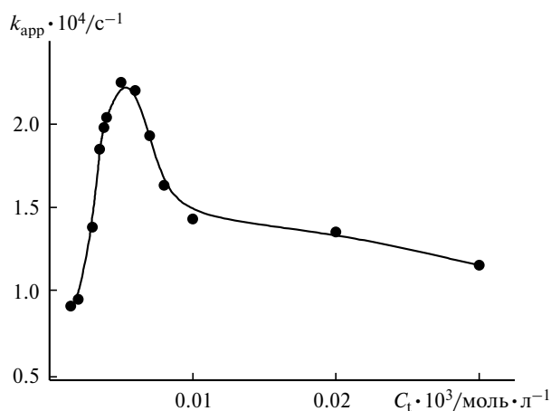
Рис. 5. Зависимость наблюдаемой константы скорости гидролиза фосфата 7 от концентрации КПАВ 3 при 25 °С, C_{\text{NaOH}} = 10^{-3} моль \cdot л ^{-1} .
