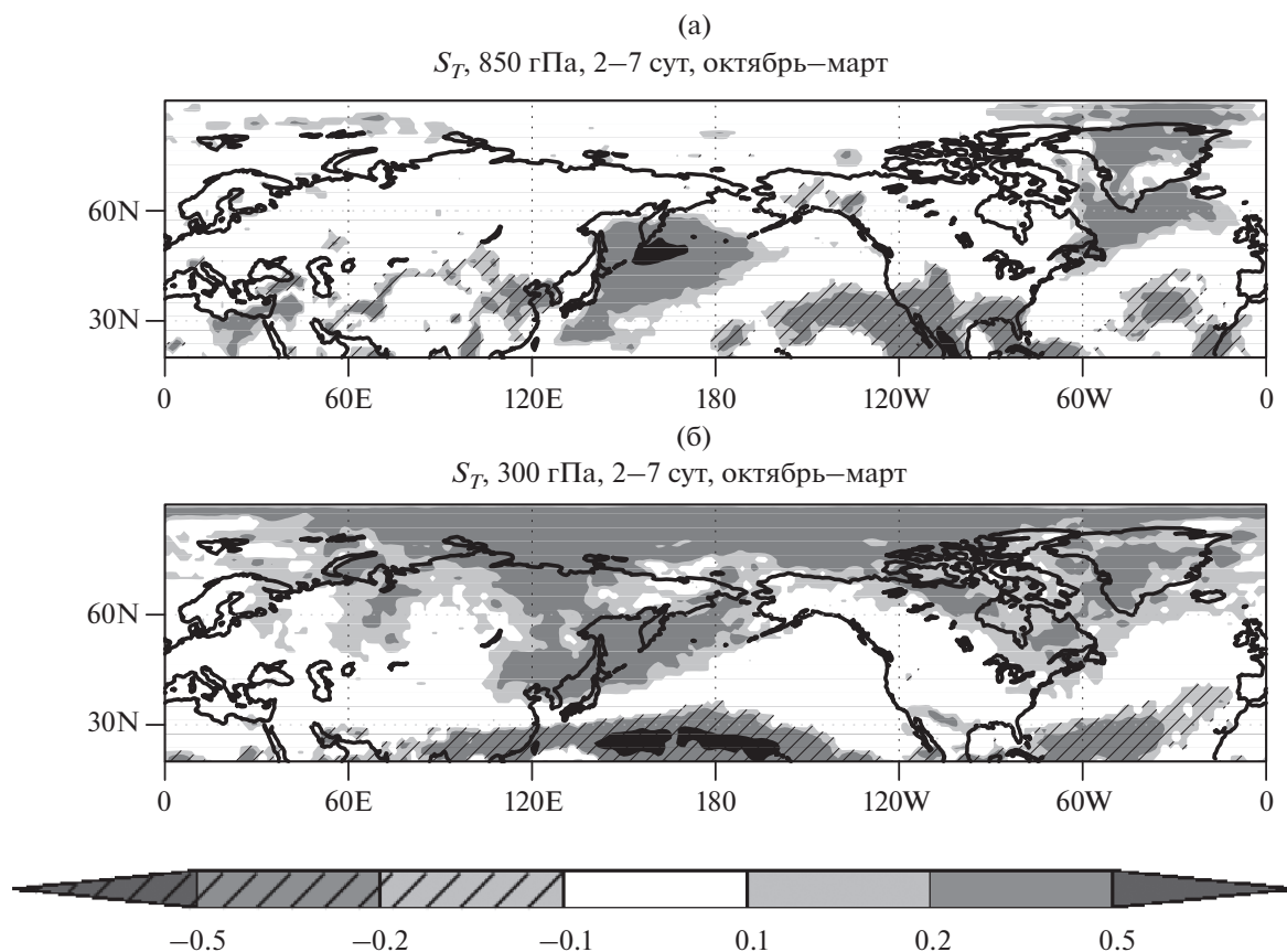
Рис. 4. Аналогично рис. 2, но для асимметрии выборочной функции распределения вероятности температуры в октябрь–марте для интервала временных масштабов 2–7 сут на уровнях 850 гПа (а) и 300 гПа (б).
