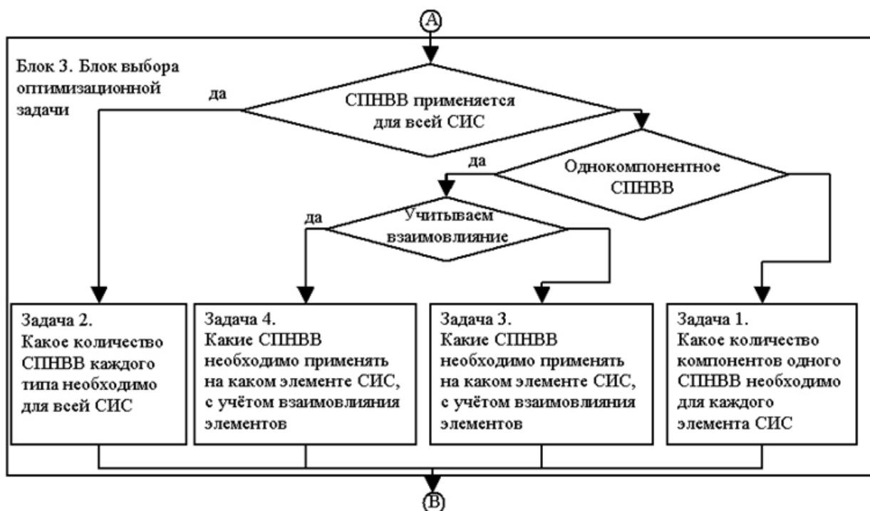
Рис. 3. Блок-схема процедуры выбора оптимизационной задачи в СППР по выбору СПНВВ для СИС
