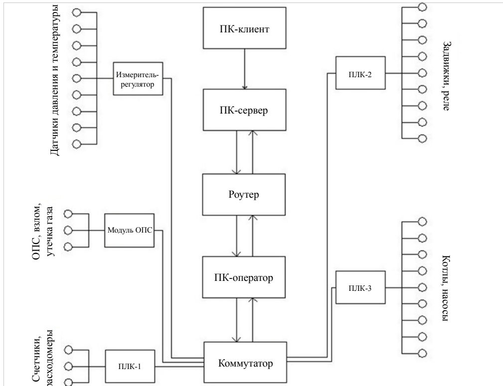
Рис. 1. Система удаленного мониторинга за работой энергетических установок
