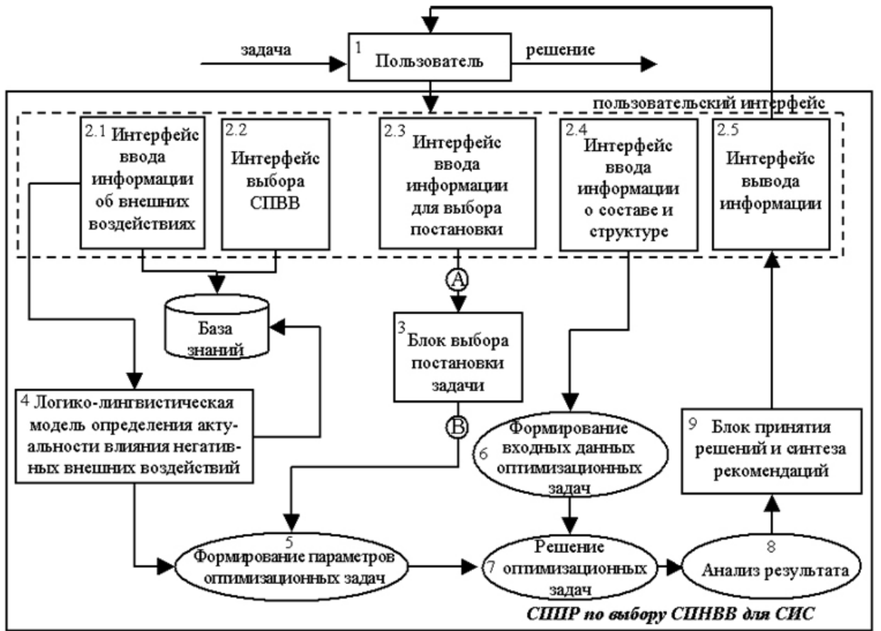
Рис. 2. Структурная модель СППР по выбору СПНВВ для СИС
