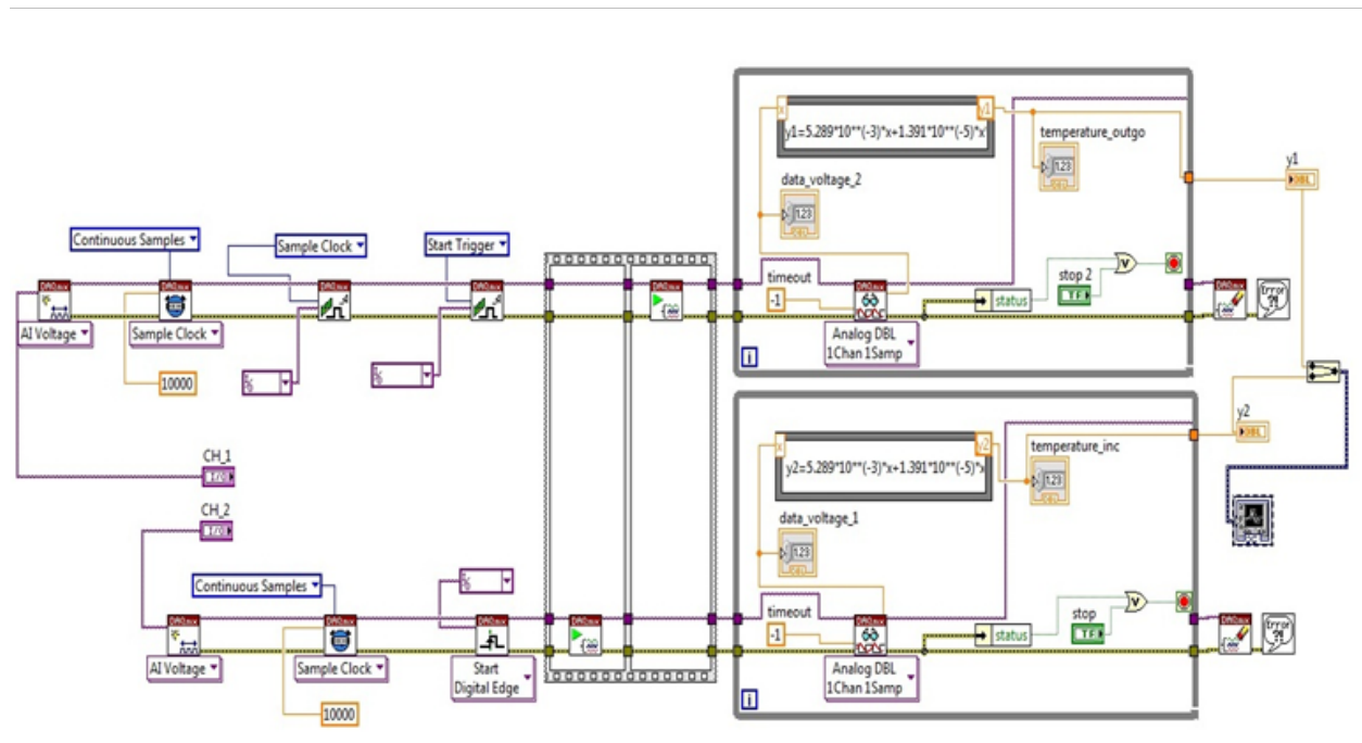
Рис. 2. Подсистема опроса термодпар прямой и обратной линий теплоносителя котельной
