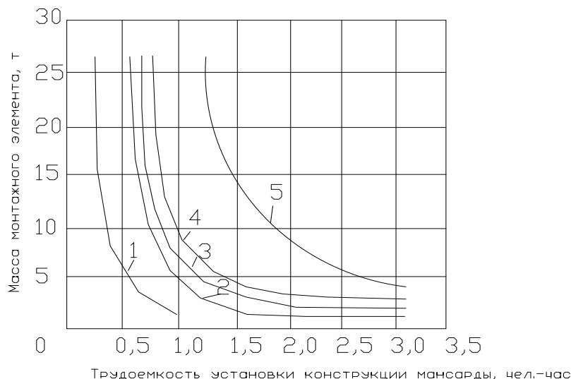
Рис. 1. График удельной трудоемкости установки монтажных модулей в зависимости от их массы: 1 – ригели и прогоны; 2 – колонны; 3 – балки; 4 – стропильные и подстропильные фермы; 5 – укрупненные блоки конструкций
