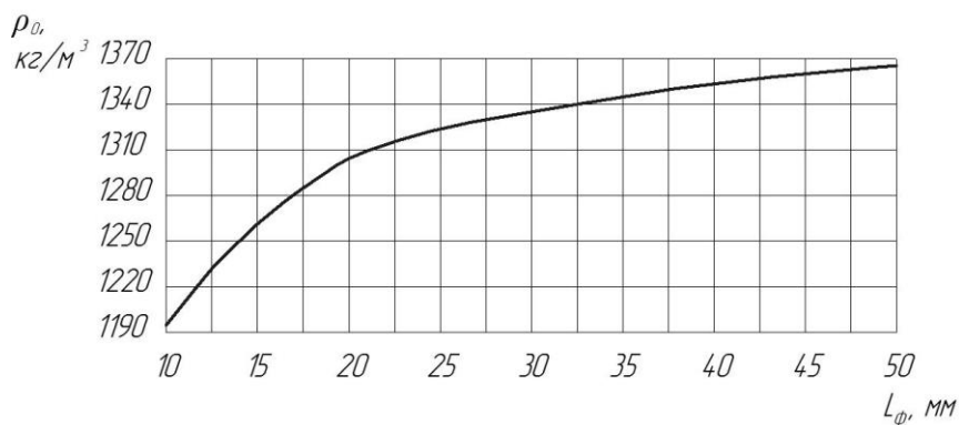
Рисунок 2 - Зависимость плотности гранул \rho_0 на выходе прессующего органа от длины L фторопластового канала при рабочем давлении P=6,85 МПа, влажности материала 31% и длины стальной части L_c = 9 мм
