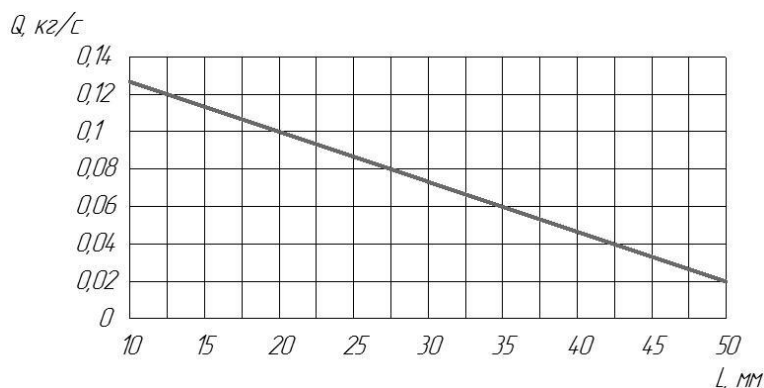
Рисунок 3 - Зависимость производительности Q гранулятора от длины L фторопластового канала при рабочем давлении P=6,85 МПа, влажности материала 31% и длины стальной части L_c = 9 мм
