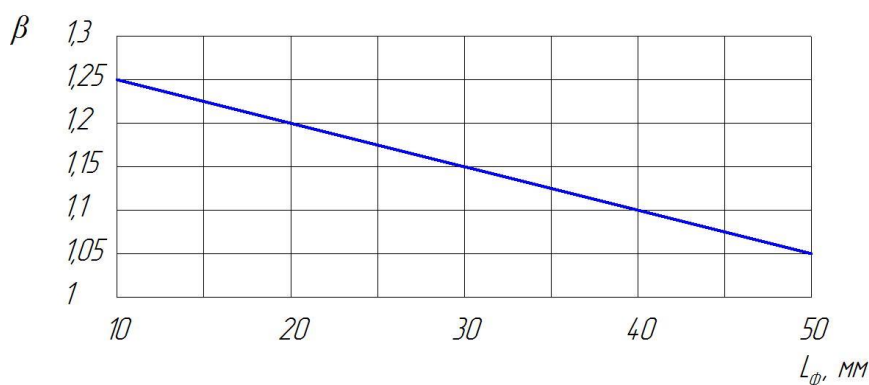
Рисунок 1 - Зависимость коэффициента линейного расширения \beta от длины L фторопластового канала при рабочем давлении P=6,85 МПа, влажности материала 31% и длины стальной части L_c = 9 мм
