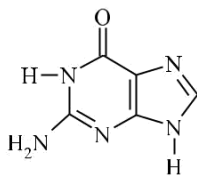
Гуанин (Г) (РНК+ДНК)
