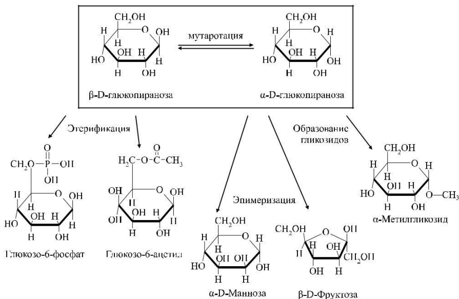
Схема химических превращений D-глюкозы
