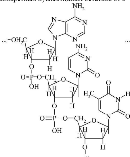
... A_{\text{д}} - C_{\text{д}} - T_{\text{д}} ... (фрагмент ДНК)
