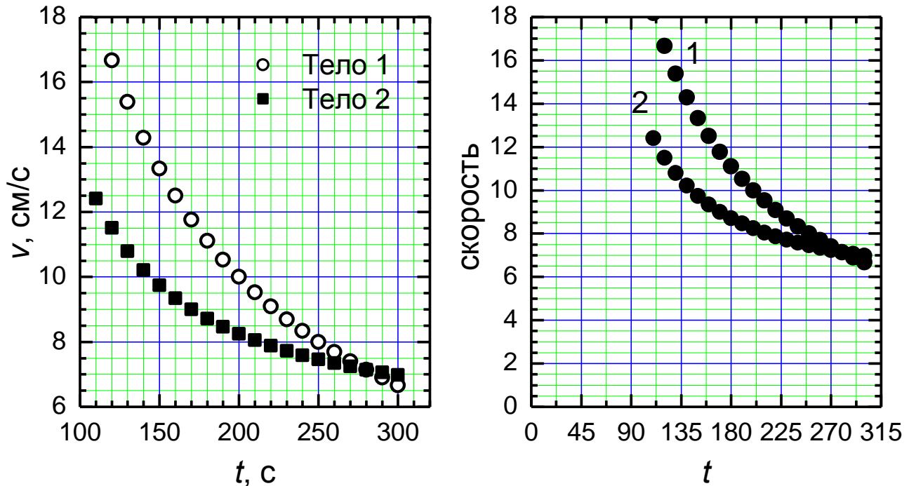
Рис. 1. Графики изменения модуля скорости v тела 1 (пустые кружки) и 2 (квадратики) со временем t .
