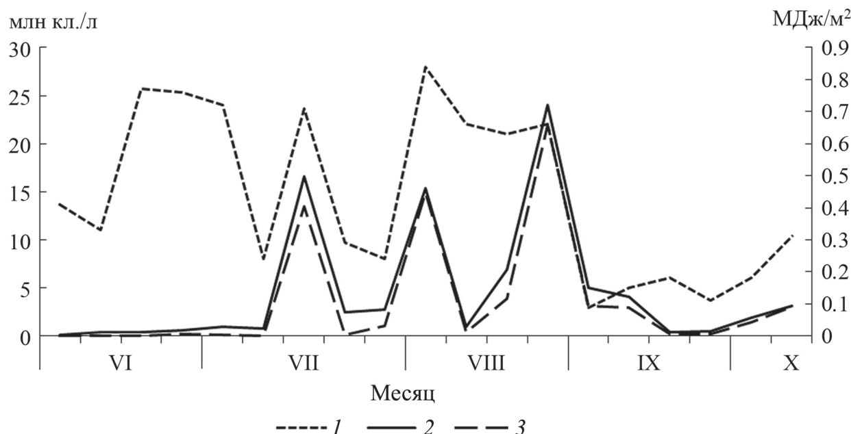
Рис. 6. Динамика суммарной солнечной радиации (МДж/м 2 ) (1), общей численности фитопланктона (2) и численности цианобактерий (3) (млн кл./л) в интегрированных пробах Волжского плеса Куйбышевского водохранилища в 2017 г.
