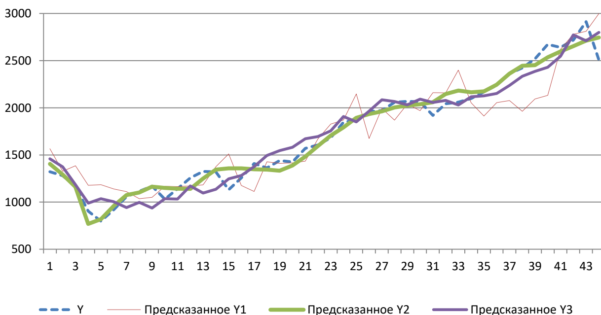
Рис.1. Фактические и предсказанные (по моделям 1,2,3) данные индекса S&P500
