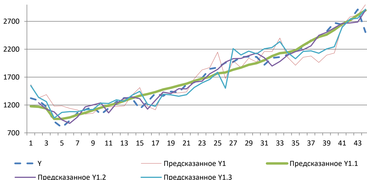
Рис.2. Фактические и предсказанные (по моделям 1, 1.1, 1.2, 1.3) данные индекса S&P500
