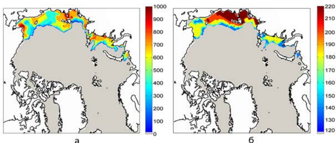
Рис. 1. (а) - Рассчитанная мощность зоны стабильности гидратов метана (в м) в условиях субаквальной мерзлоты для мелководных шельфов арктических морей; (б) – положение верхней границы зоны стабильности под морским дном (в м).
