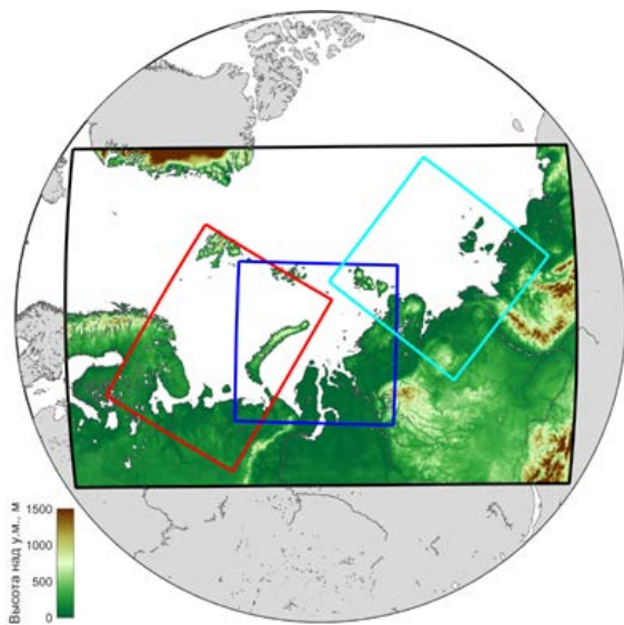
Рис. 1. Предварительная схема областей моделирования. Черный прямоугольник показывает «базовую» область с шагом сетки ~13 км, красный, синий и бирюзовый – вложенные области моделирования с шагом сетки ~3.3 км соответственно для Баренцева моря, Карского моря и моря Лаптевых.
