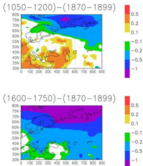
Рис. 2. Среднегодовая приземная температура, осредненная по указанным временным интервалам.
