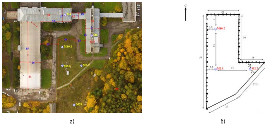
Рис. 1. Схема расположения мачт (а) и нижней (наземной) наблюдательной площадки (б) Геофизической обсерватории ИМКЭС СО РАН.
