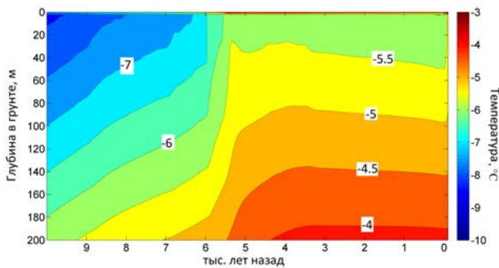
Рис. 2. Рассчитанная среднегодовая температура грунта за последние 10 тыс. лет для региона Ямала.
