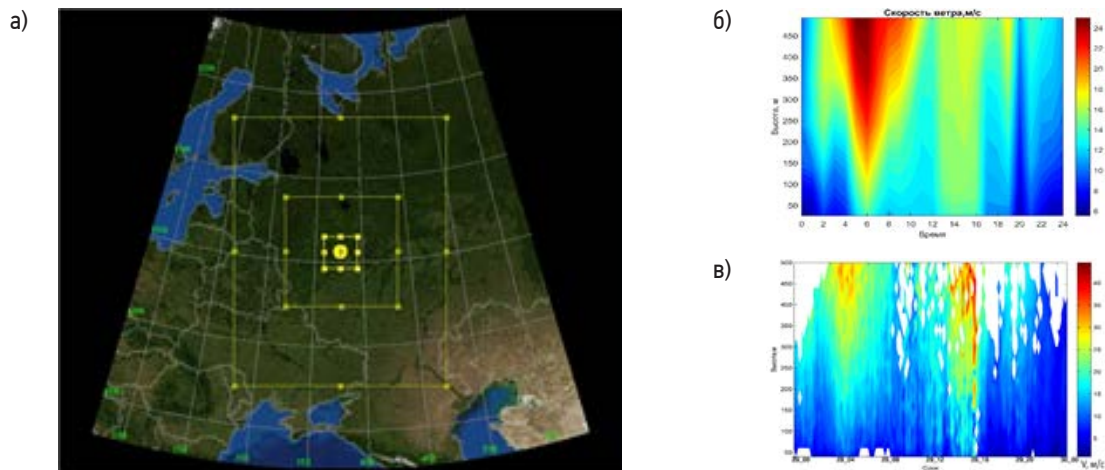
Рис. 1. Границы области моделирования (а), результат моделирования скорости ветра в нижнем 500-метровом слое в г. Москвы (б) и данные содара MODOS (в).
