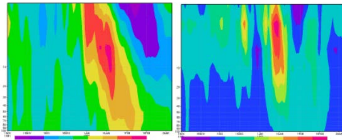
Рисунок 1. Аномалии температуры полярной стратосферы в ноябре 1991 - феврале 1992 года по данным модели ПЛАВ (слева) и реанализа ERA-Interim (справа). Можно наблюдать положительную аномалию температуры в районе 16 января.
