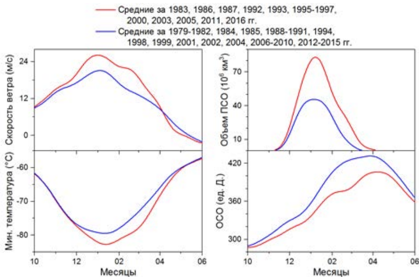
Рис. 2. Внутригодовой ход скорости зонального ветра на 60^\circ с.ш. и минимальной температуры в области 50^\circ – 90^\circ с.ш. на высоте 50 гПа (~20 км), объема ПСО в области 60^\circ – 90^\circ с.ш. и ОСО в области 63^\circ – 90^\circ с.ш. в среднем за годы с регистрируемыми озоновыми аномалиями (красные кривые) и в их отсутствии (синие кривые).
