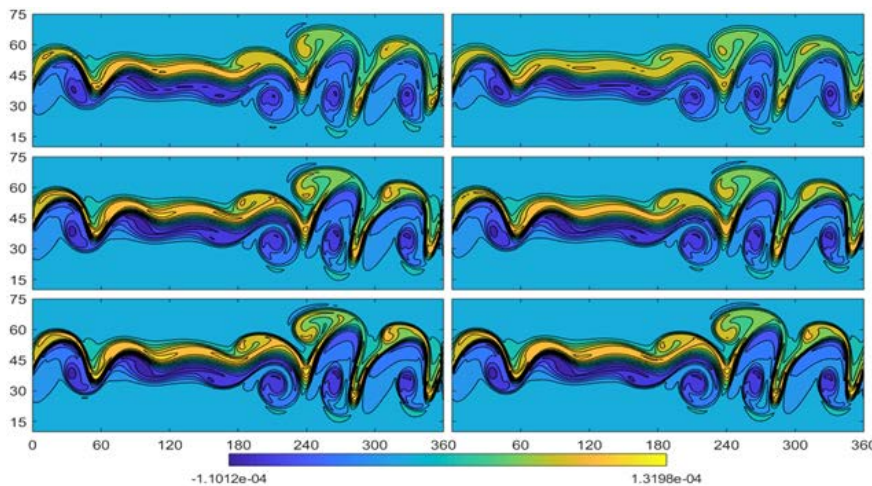
Рисунок 3. Поле относительные завихренности на момент T=144 ч модельного времени. Левый столбец – расчет с использованием редуцированной сетки с разнесением переменным, правый столбец – без разнесения переменных. Коэффициент редукиции сетки \alpha=0.5 . Разрешение сетки до применения редукиции (сверху вниз) – 256 \times 128 , 384 \times 192 , 512 \times 256 .
