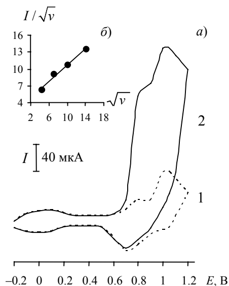
Рис. 2. а) Циклические вольтамперограммы, полученные на ХМЭ на основе пленки RuO-RuCN в отсутствие (1) и в присутствии 1 \cdot 10^{-2} моль/л гентамицина (2) на фоне 0.01 М H_2SO_4 ; б) зависимость I/\sqrt{v} от \sqrt{v} при окислении гентамицина на ХМЭ
