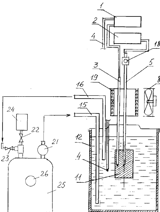
Рисунок 8.2 Схема экспериментальной установки
