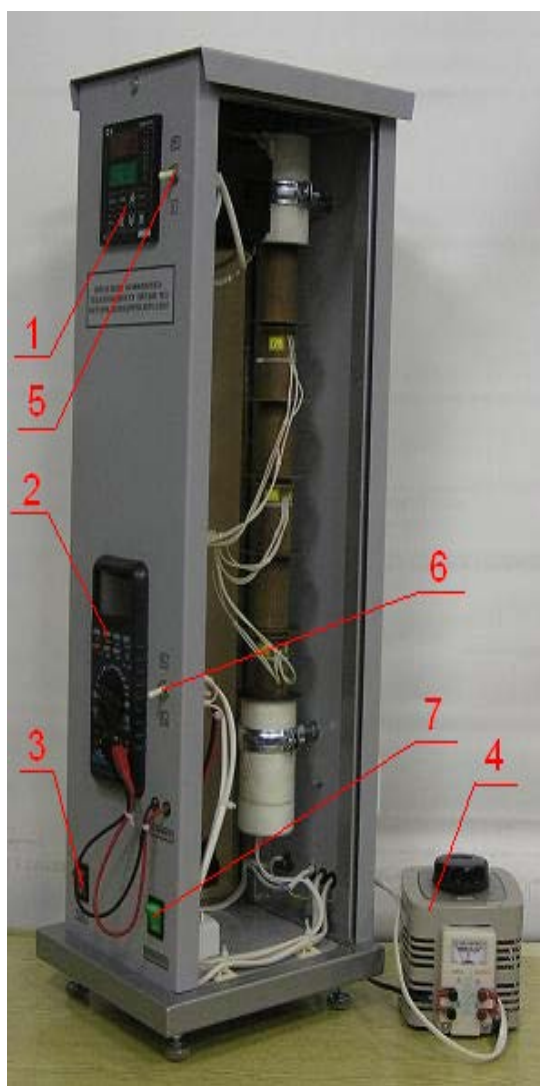
Рисунок 10.1 Экспериментальная установка
