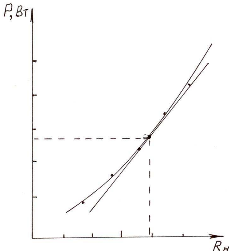
Рисунок 7.1 Примерный вид экспериментальной зависимости P = f(R_n)
