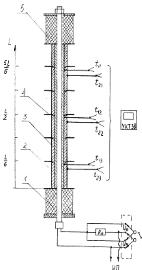
Рисунок 10.2 Схема экспериментальной установки
