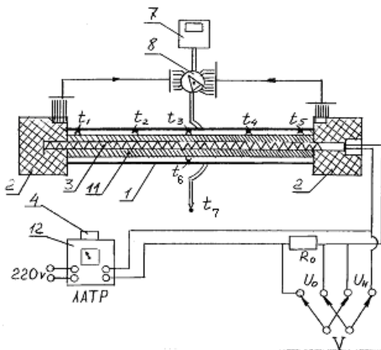
Рисунок 6.2 Схема экспериментальной установки
