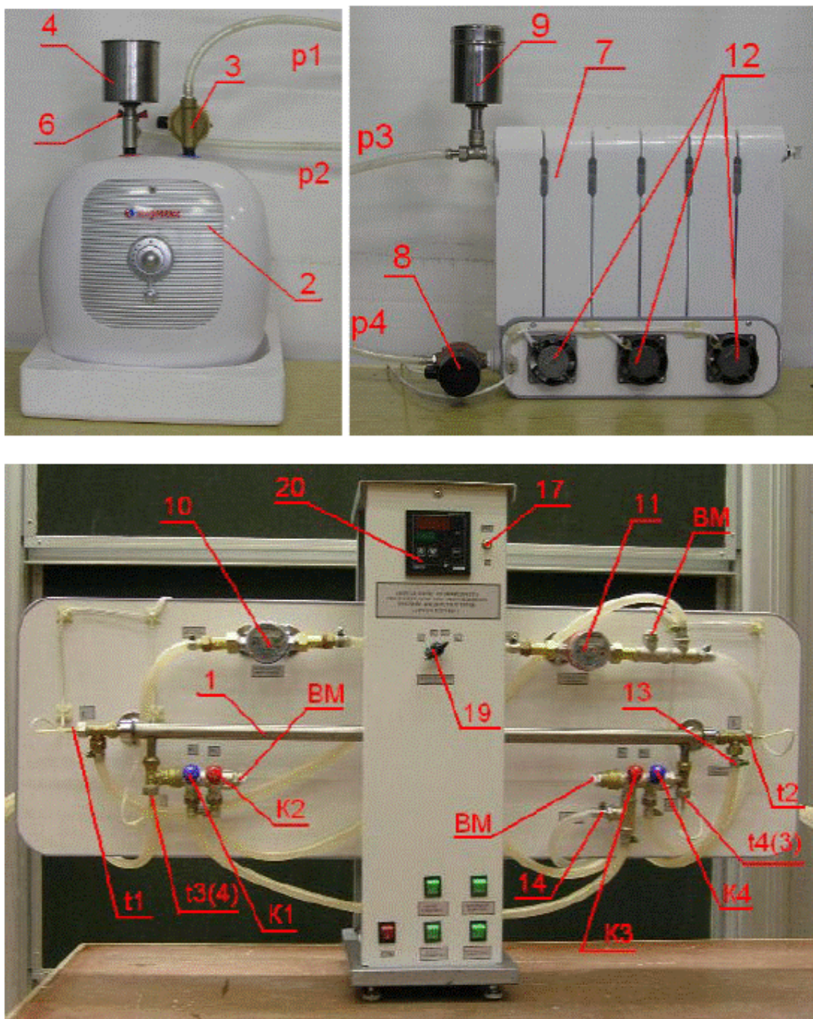
Рисунок 11.3 Внешний вид стенда
