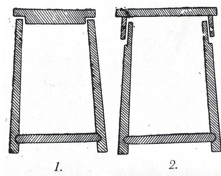
Рис. 1. Конструкция паря: 1) крышка вставляется в парь; 2) крышка надевается на парь
