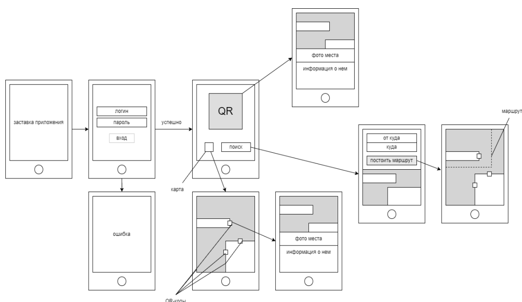
Рис. 5. Схема работы приложения
