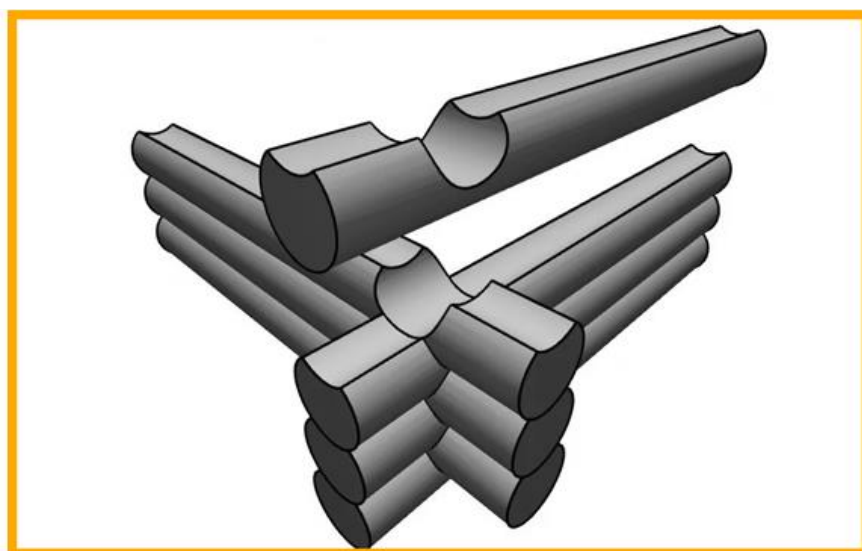
Рис. 2. Рубка «в обло»
