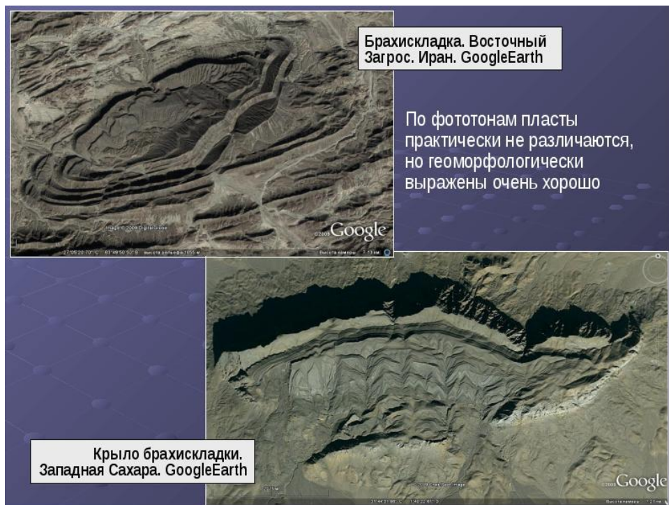
Рис. 2. Складчатые структуры на аэрофотоснимках
