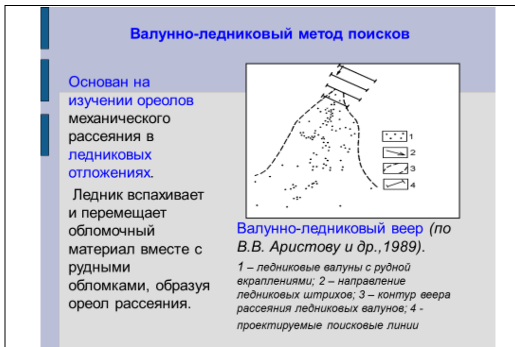
Рис. 12. Валунно-ледниковый метод поисковых работ
