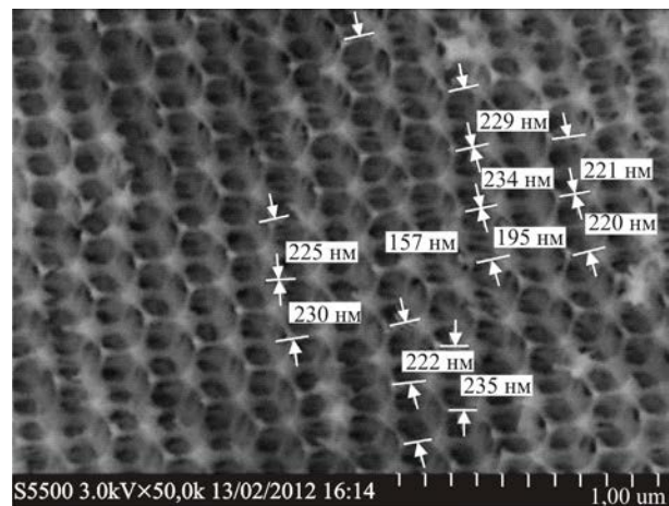
Рис. 1. Образец 1 инверсного опала с размерами пор (224 \pm 15) нм.
